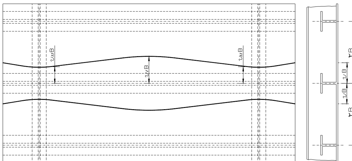
شکل ۶-۳- عرض موثر ورقه رویه
