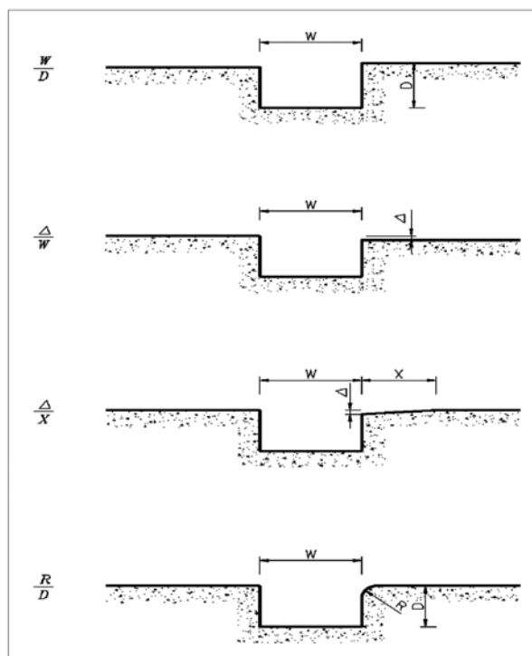
شکل ۳-۱۲ - هندسه شیار
