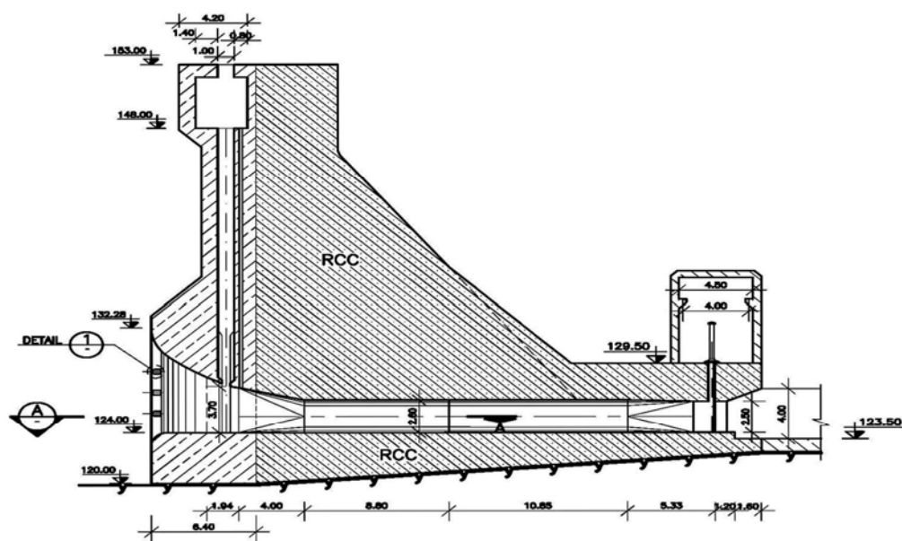
مقطع طولی تخلیه کننده عمقی شماره ۱ سد جگین
