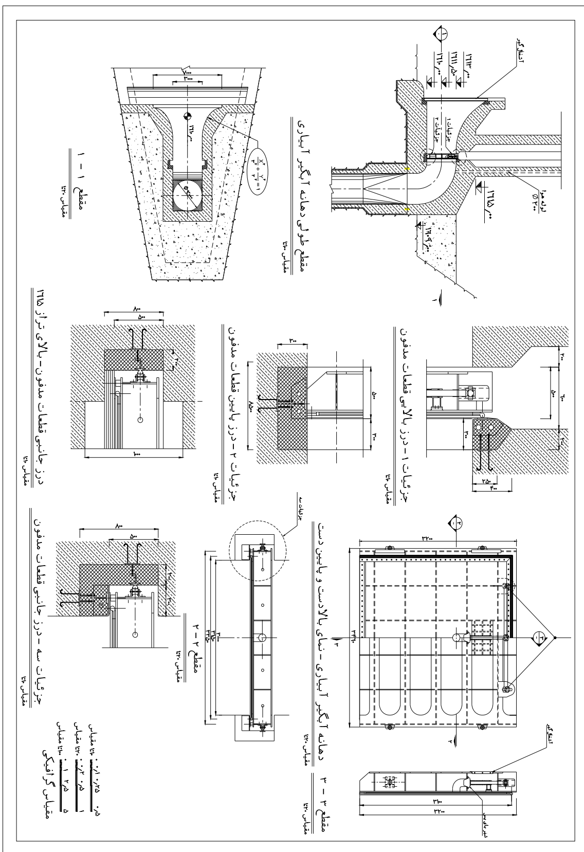
شکل ۴-۲۱- درپشه رأس تخلیه کننده عمقی سد تالوار
