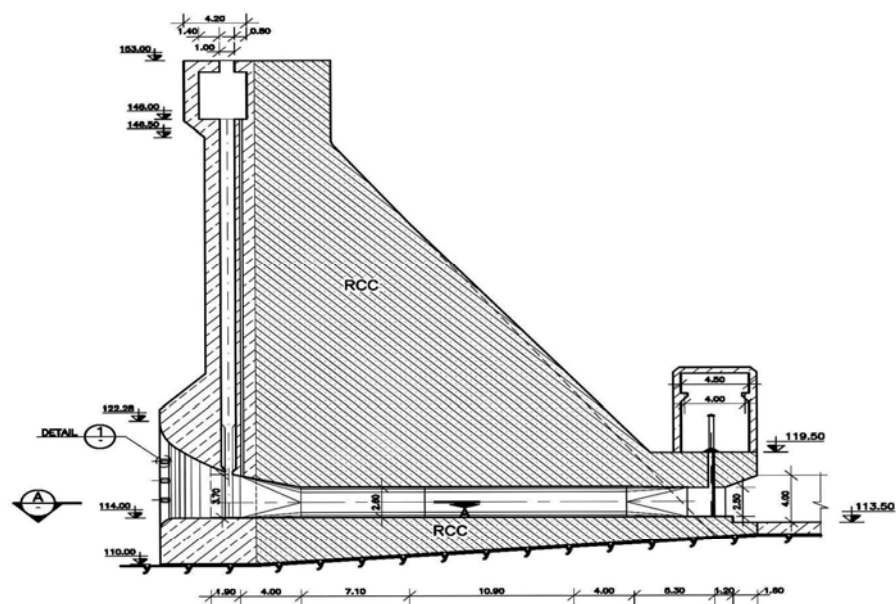
مقطع طولی تخلیه کننده عمقی شماره ۲ سد جگین
