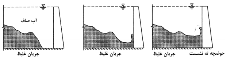
شکل ۳-۲- حرکت جریان غلیظ در مجاورت بدنه سد
