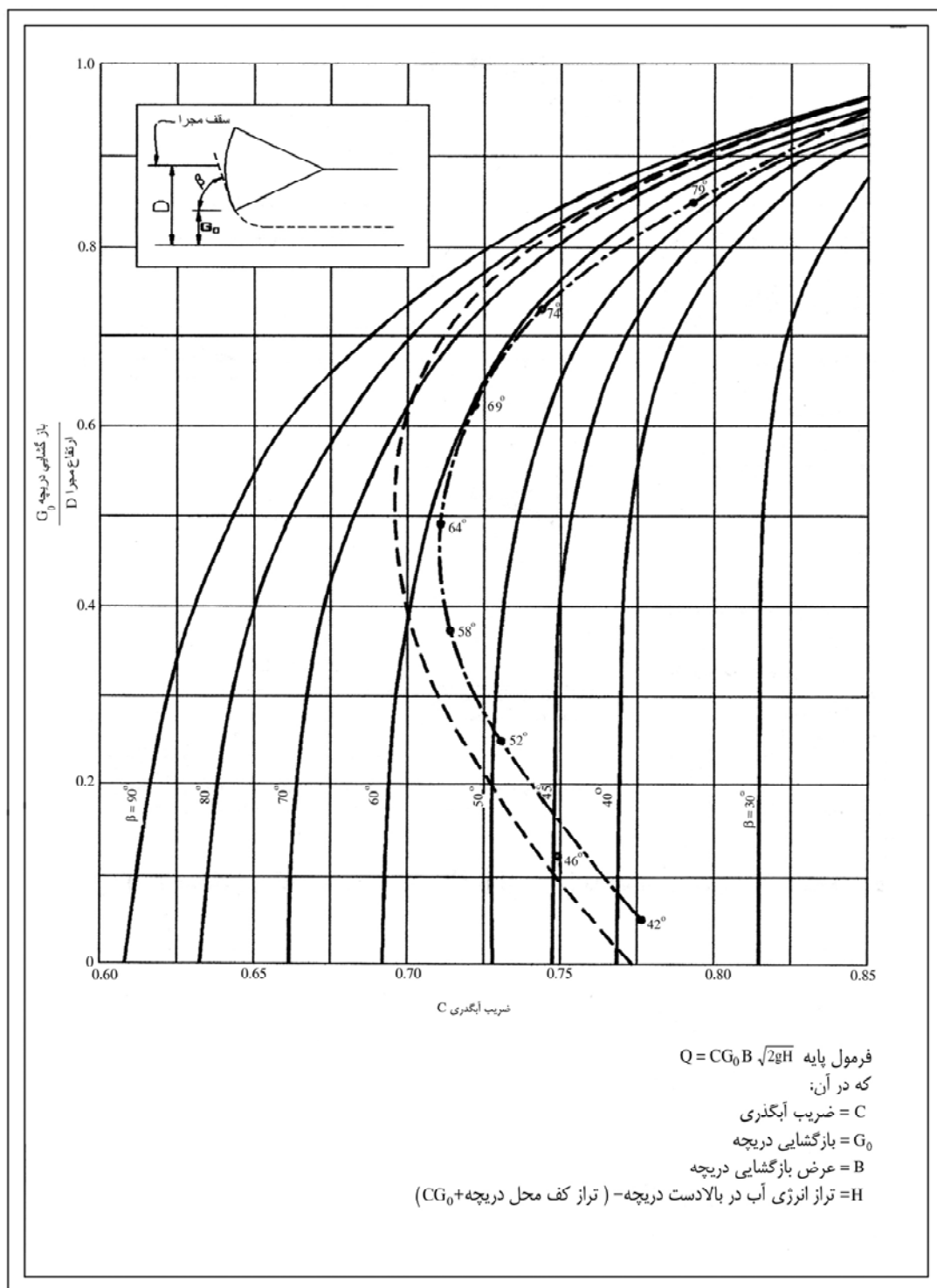
شکل ۳-۹- ضریب آبگذری دریچه قطاعی [۷]
