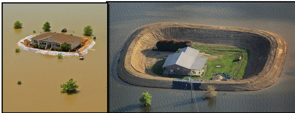
شکل ۳-۴- نمونه‌ای از خاکریزها و سکوه‌های شیروانی خاکی اجرا شده در زمان وقوع سیلاب
