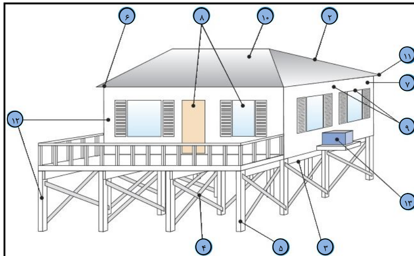
شکل ۳-۱۶- نکات قابل توجه در طراحی و ساخت در کنار سواحل (برای شماره‌های موجود در شکل توضیحات مربوط در متن راهنما وجود دارد) [۴۸]
