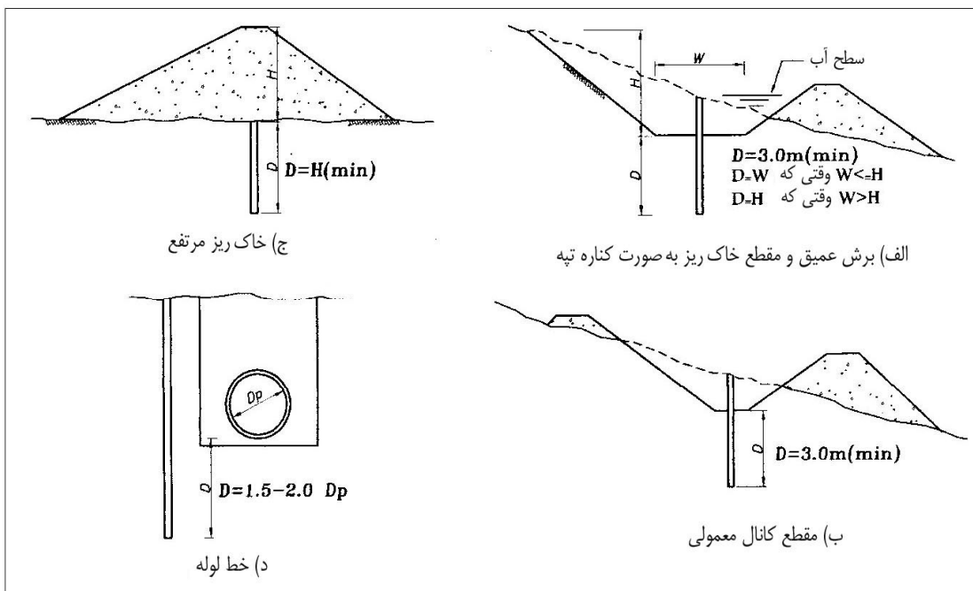
شکل ۴-۲ عمق پیشنهادی گمانه‌ها برای سازه‌های نواری [۱]
