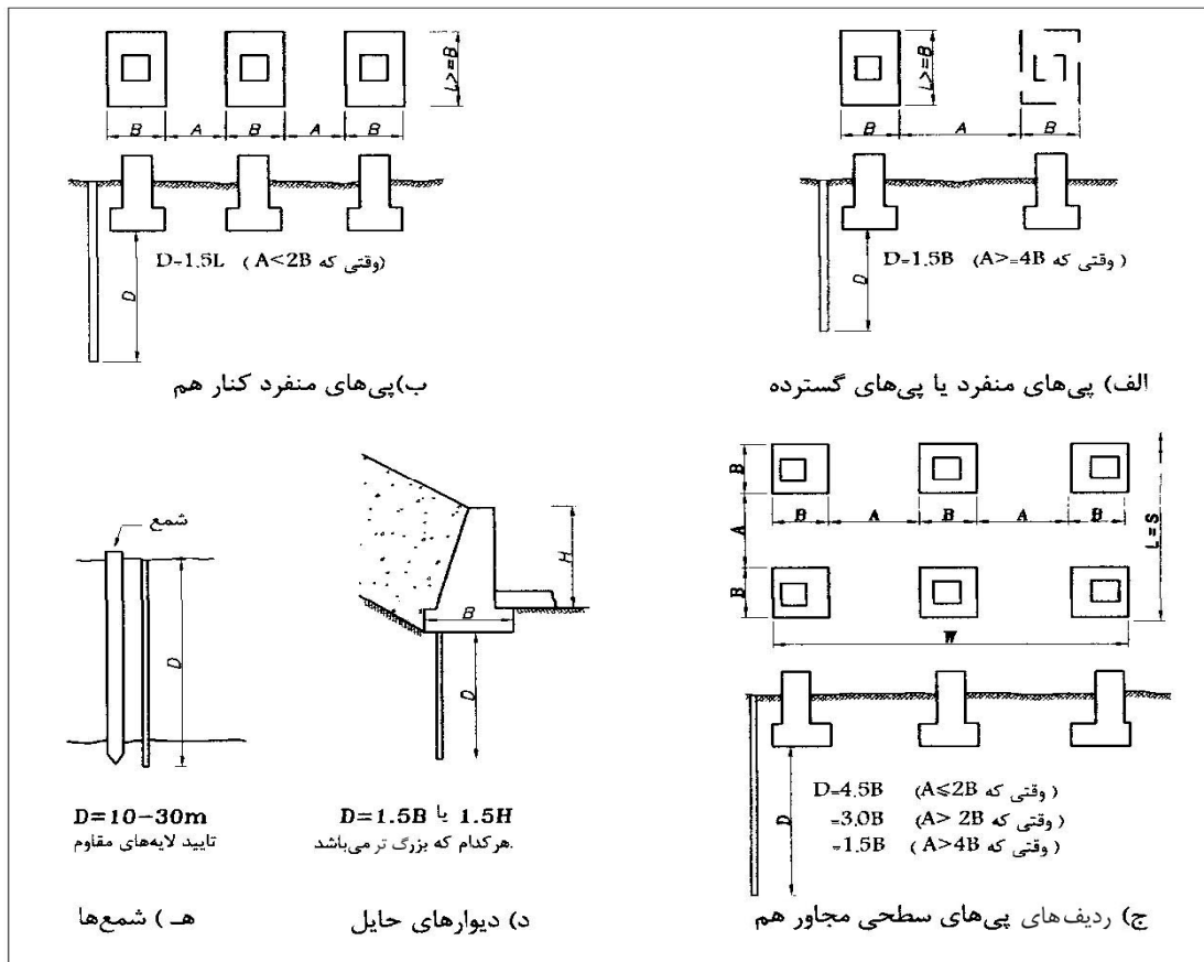
شکل ۴-۱ عمق پیشنهادی گمانه‌ها برای پی‌های نقطه‌ای [۱]
