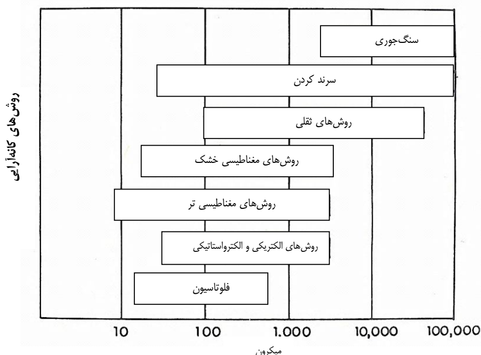
شکل ۱-۲- محدوده ابعادی موثر در فرآیندهای مختلف کانه‌آرایی
