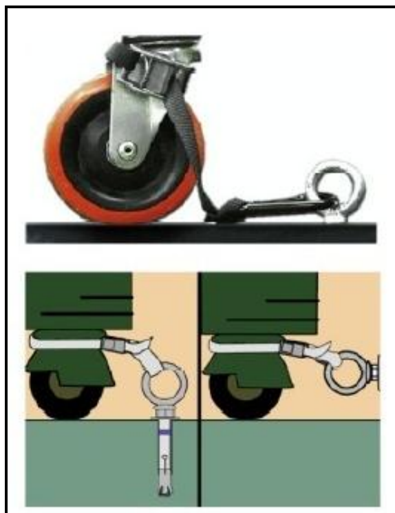
شکل ۴-۱۸- استفاده از حایل برای مهار وسیله چرخ‌دار
