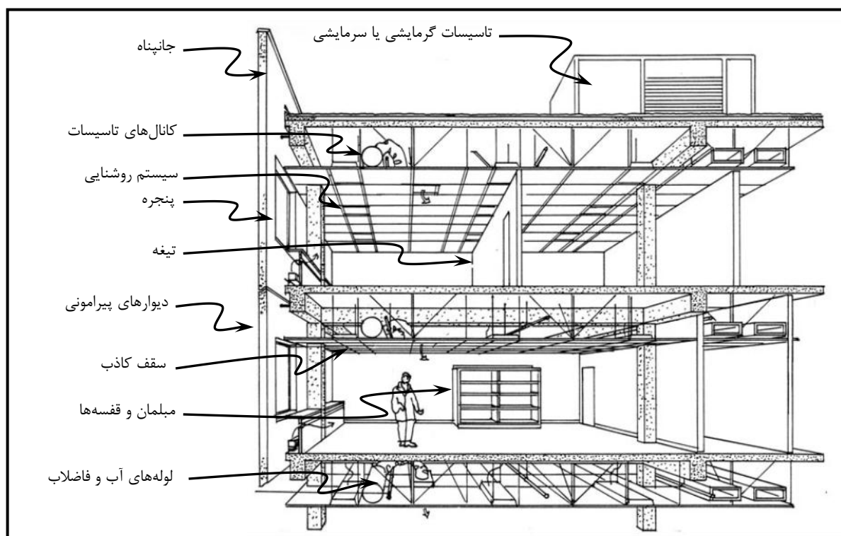
شکل ۴-۱- اجزای غیرسازه‌ای ساختمان به صورت شماتیک
