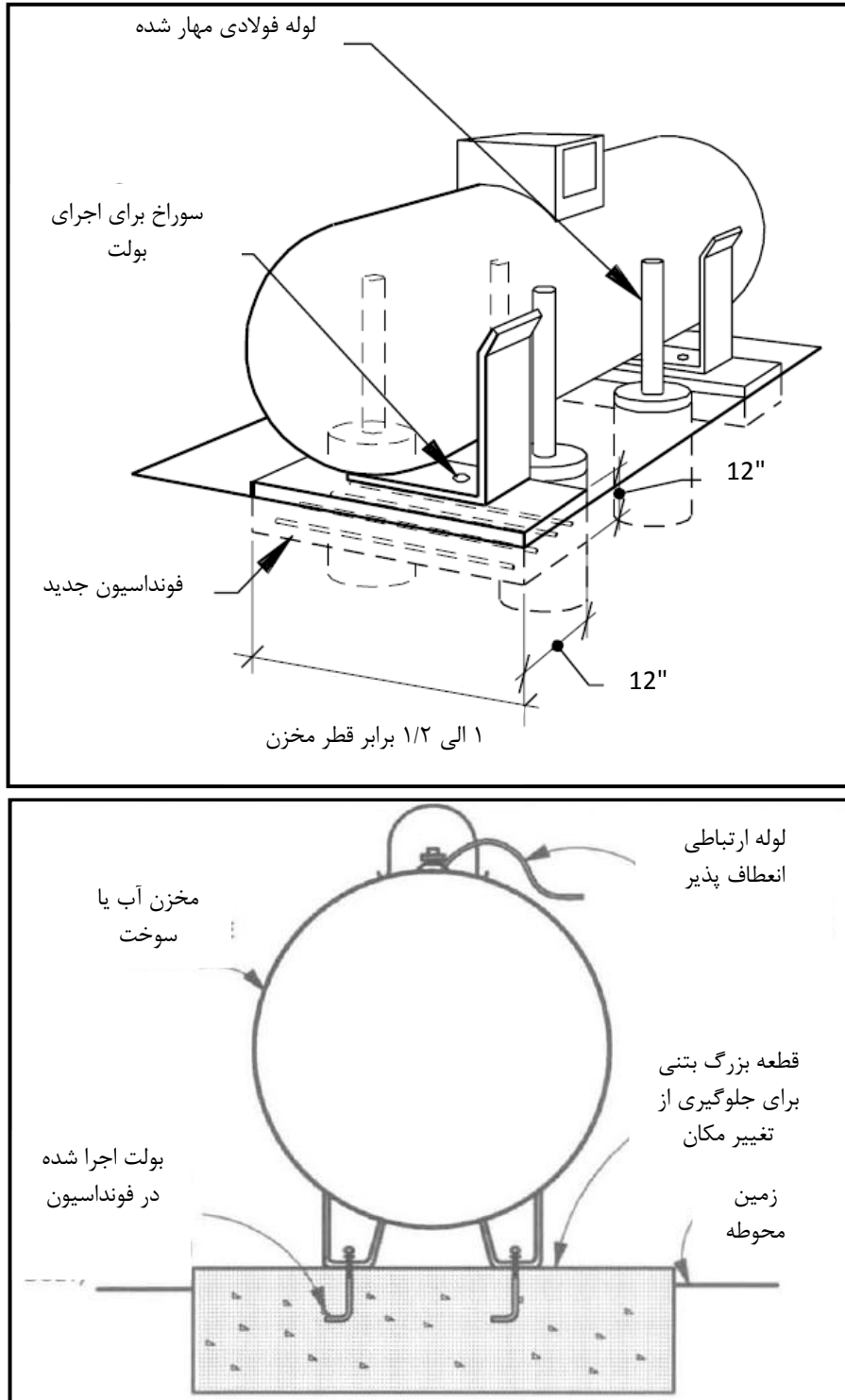
شکل ۴-۲۴- نحوه مهار مخزن آب یا سوخت
