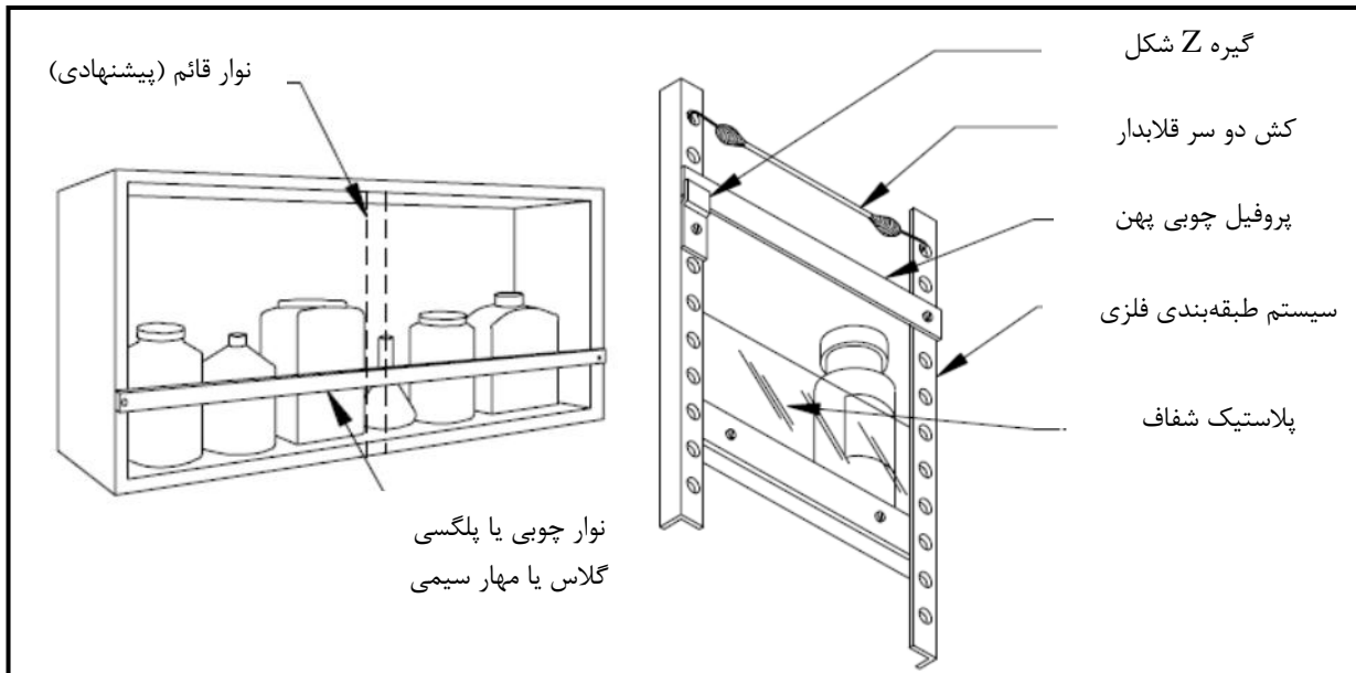
شکل ۴-۱۹- جزئیات اجرایی مهر تجهیزات خطر آفرین
