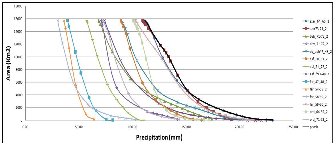
شکل ۷-۶- منحنی‌های سطح - عمق بارش برای تداوم دو روزه
