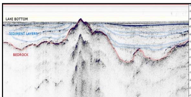
شکل ۴-۴- تصویر حاصله از داده‌های ثبت شده نیمرخ‌بردار بستر دریا
