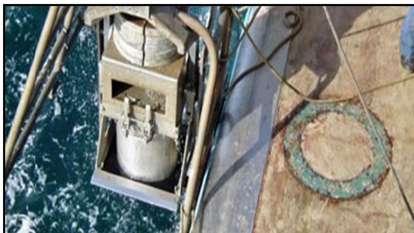
شکل ۲-۶- مغزه گیر Haja
