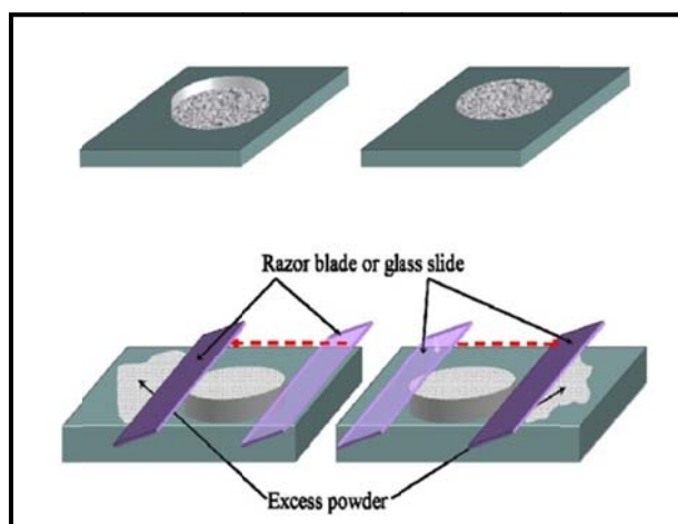
شکل ۳-۱۰- صاف نمودن سطح نمونه
