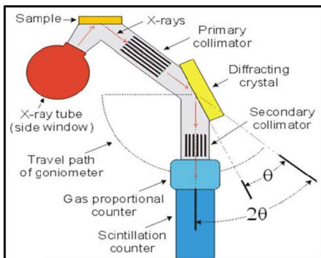
شکل ۳-۱۱- شماتیکی از نحوه انتقال اشعه ایکس در دستگاه X-Ray
