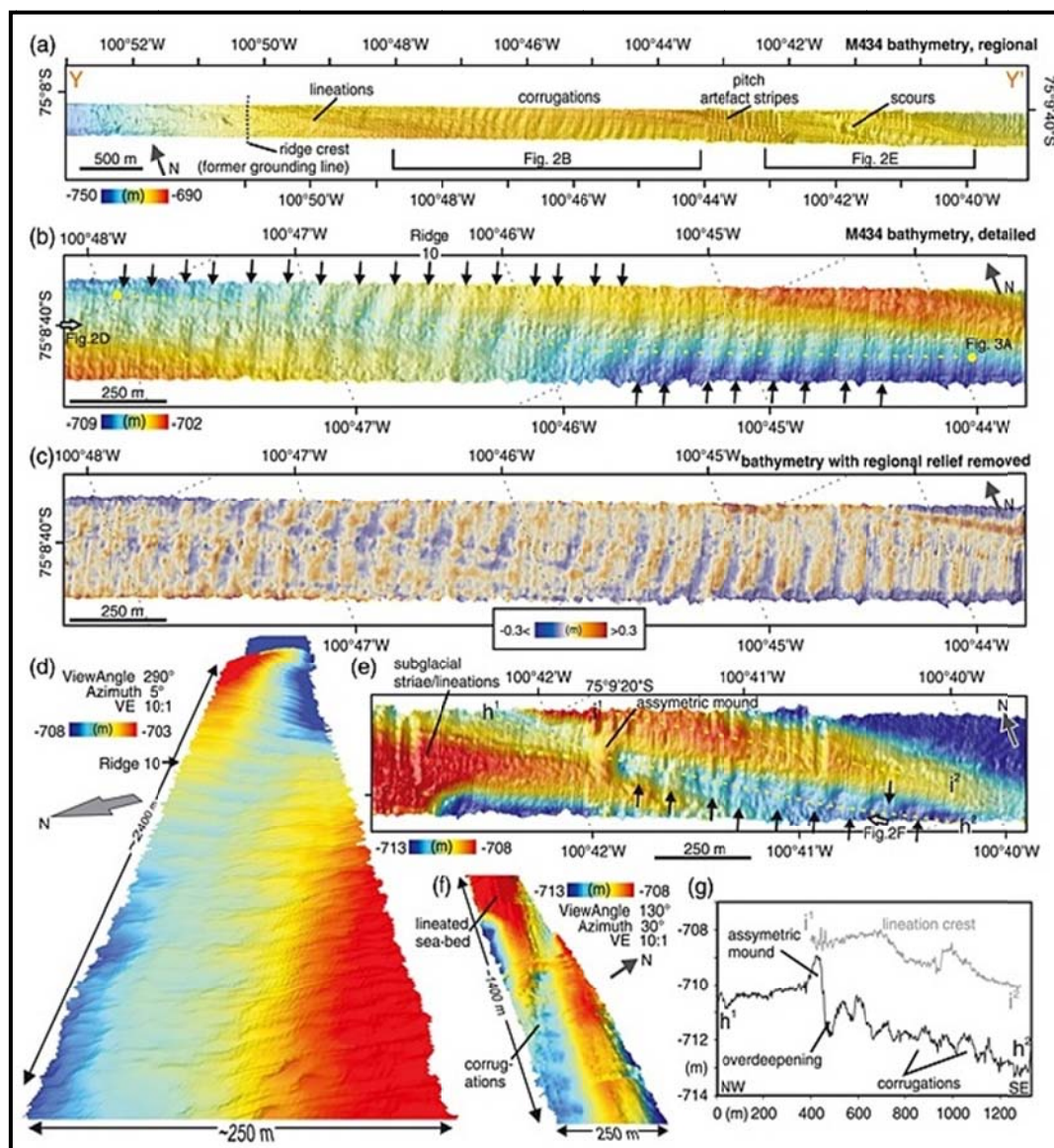
شکل ۱-۴- نتایج عمق سنجی (a) برداشت نوار عرضی، (b) مشخصات بستر بر اساس شیارها (فلش‌ها)، (c) بستر شناسی بر اساس حذف پستی و بلندی‌ها، (d) نمایش بستر ۳ بعدی بر اساس شیارها (بر اساس فلش سفید رنگ در تصویر b و e و f) مشخصات بستر شناسی بر اساس شاخص‌ها، (g) توپوگرافی بستر بر اساس مناطق مسطح
