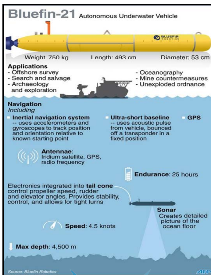
شکل ۴-۲۰- مجموعه‌ای از قطعات ربات زیردریایی خودکار
