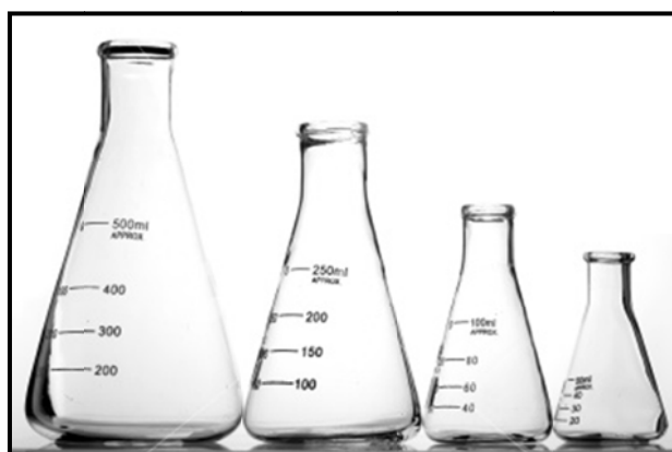
شکل ۳-۱۹- فلاسک ارلن
