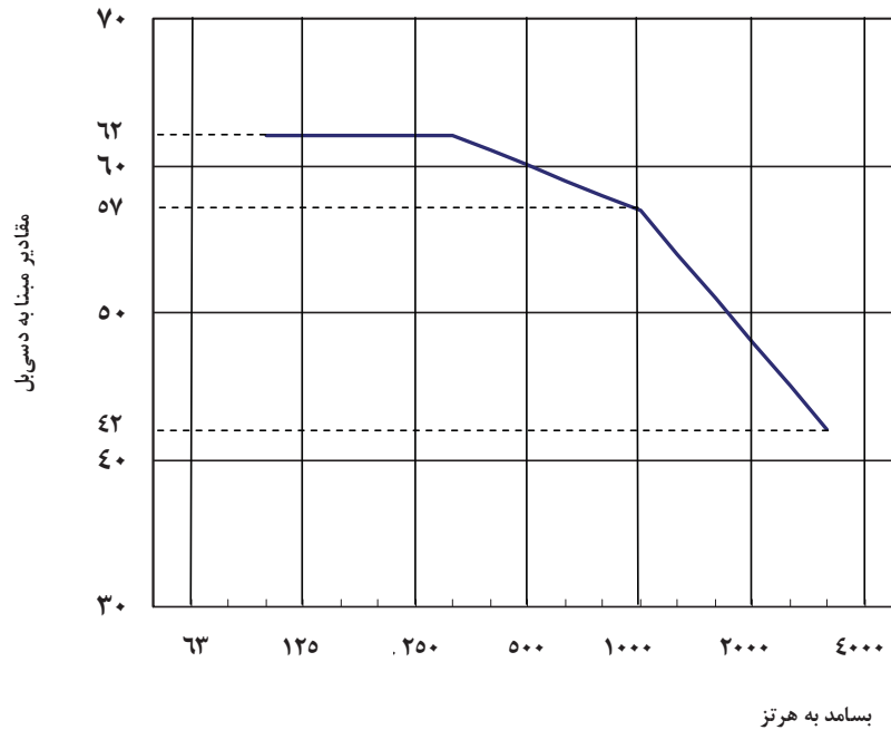
شکل ۱۸-۱-۳-۶: نمودار مقادیر مینا برای صدای کوبه‌ای، در بندهای یک‌سوم‌هنگامی
