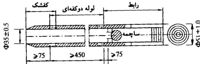
شکل شماره ۲- نمونه گیر دوکفه‌ای (ارقام برحسب میلیمتر)
