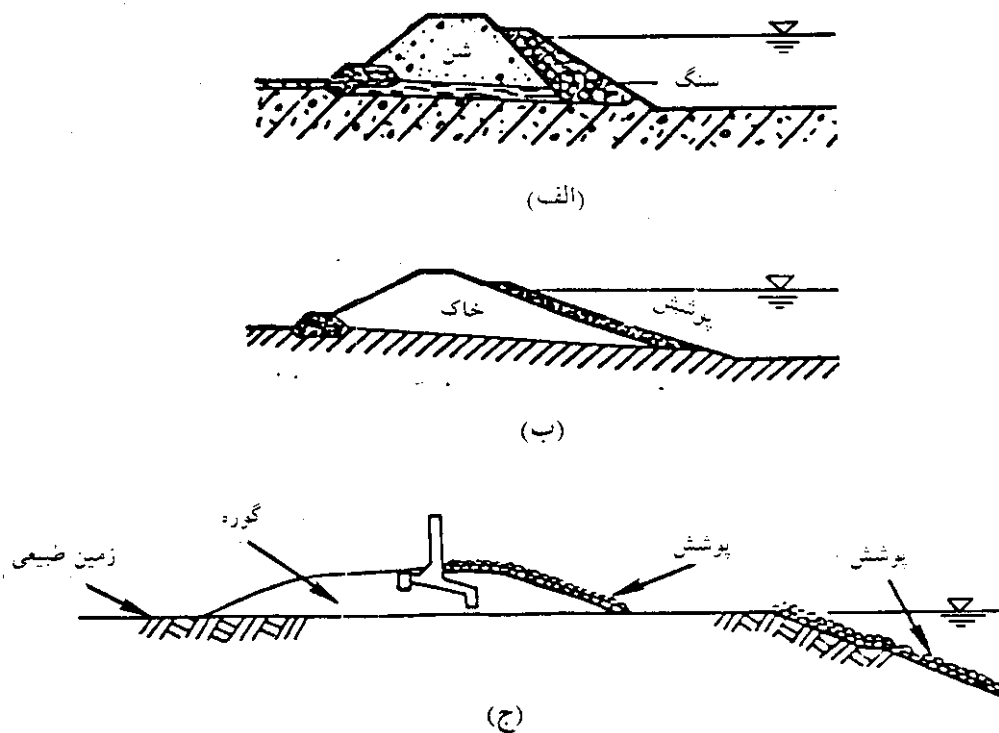
شکل ۴-۹- چند نوع گوره همگن با پوششهای محافظ مختلف
