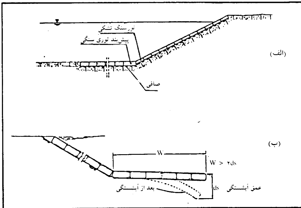
شکل ۴-۱۰- الف - تور سنگی تشکی پیش بنددار برای حفاظت شیروانی گوره و کناره رودخانه ب - تغییر شکل تور سنگ بعد از آبستگي
