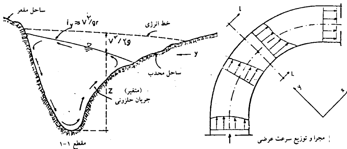
شکل ۴-۲۰- اضافه ارتفاع تراز سطح آب ناشی از جریان در خم رودخانه
