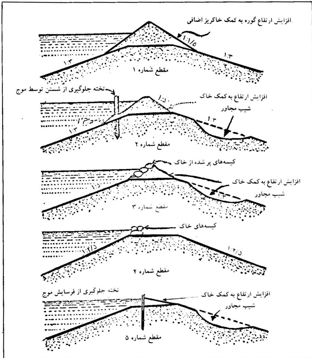
شکل ۳-۵- روشهای جلوگیری از سرریز آب در هنگام جریان سیل (روشهای مختلف بزرگسازی اضطراری گوره)
