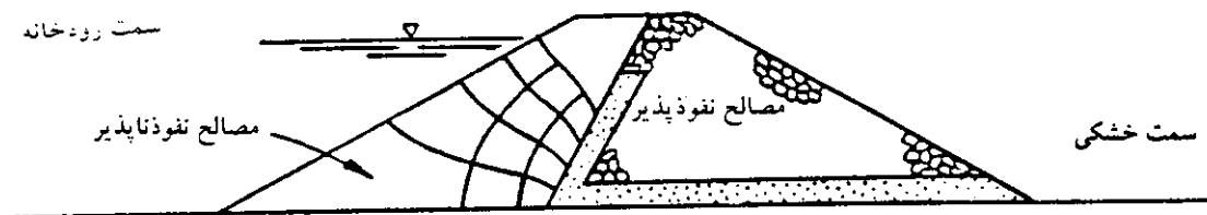
شکل ۴-۸- لایه زهکش مایل در حد فاصل مصالح نفوذناپذیر و نفوذپذیر
