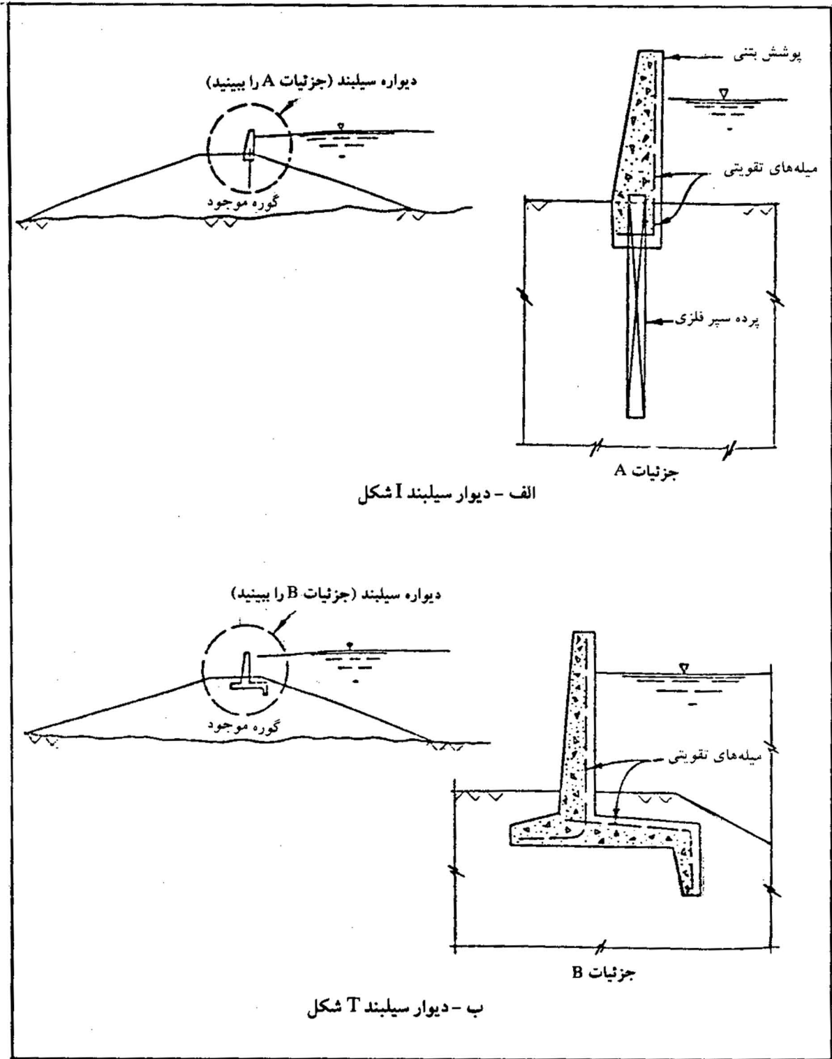
شکل ۵-۲ - بزرگسازي گوره به کمک دیوارهای سیلبنده
