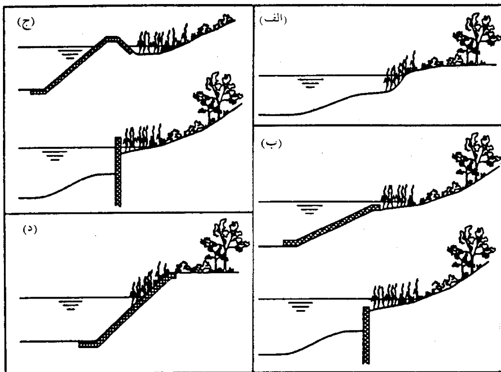
شکل ۴-۱۱- نمونه‌هایی از پوششهای حفاظتی طبیعی و طبیعی - سازه‌ای
