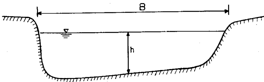
شکل ۳-۵- مقطع ساده (غیر مرکب) یک رودخانه
