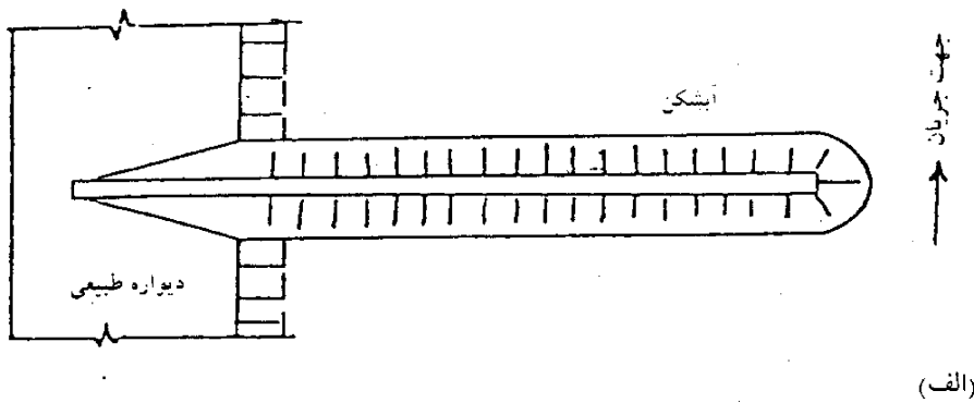
شکل ۴-۱۲- کاربرد آبشکن برای مهار فرسایش و اصلاح مسیر
