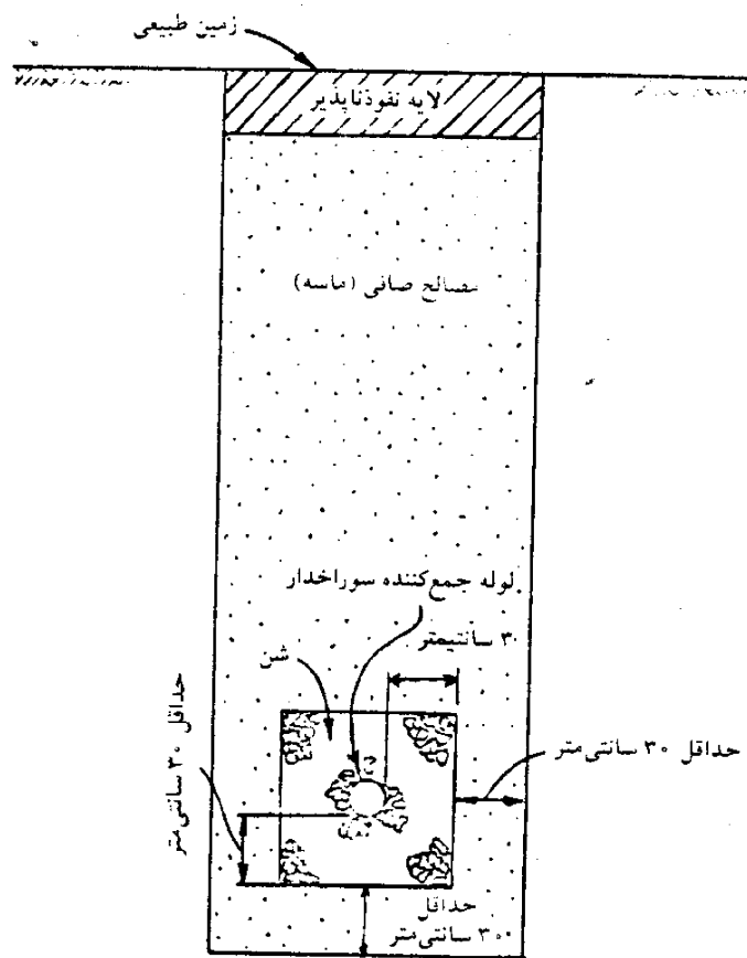
شکل ۴-۴- ترانشه زهکشی پنجه با استفاده از لوله جمع کننده در کف ترانشه
