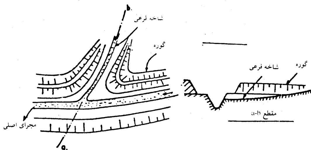
شکل ۴-۱۵- گوره فرعی در امتداد شاخه فرعی
