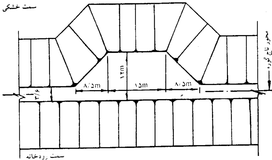
شکل ۵-۵- محل دورزدن در مسیر جاده دسترسی روی تاج گوره
