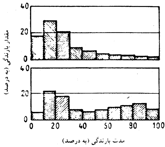
شکل ۱-۳- نمونه‌هایی از نمودار بی‌بعد شدت رگبارها
