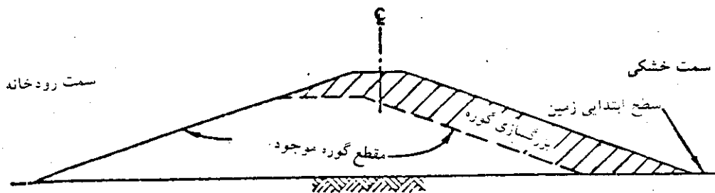
شکل ۱-۵-۱ - بزرگسازی گوره به وسیله خاک، الف - بزرگسازی در سمت رودخانه ب - بزرگسازی در دو طرف ج - بزرگسازی در سمت خشکی
