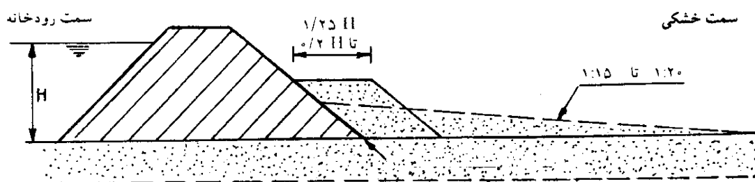
شکل ۲-۴- احداث پله (سکو) در پشت گوره به منظور حفظ پایداری و جلوگیری از
