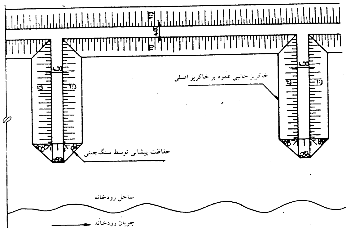
شکل ۴-۱۴- گوره آبشکن (حفاظت گوره اصلی باگوره آبشکن)
