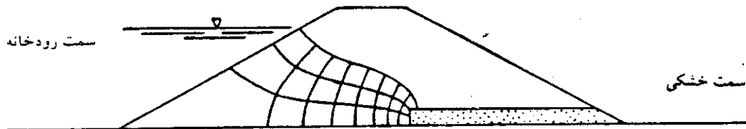
شکل ۴-۷- زهکش افقی در سمت خشکی گوره
