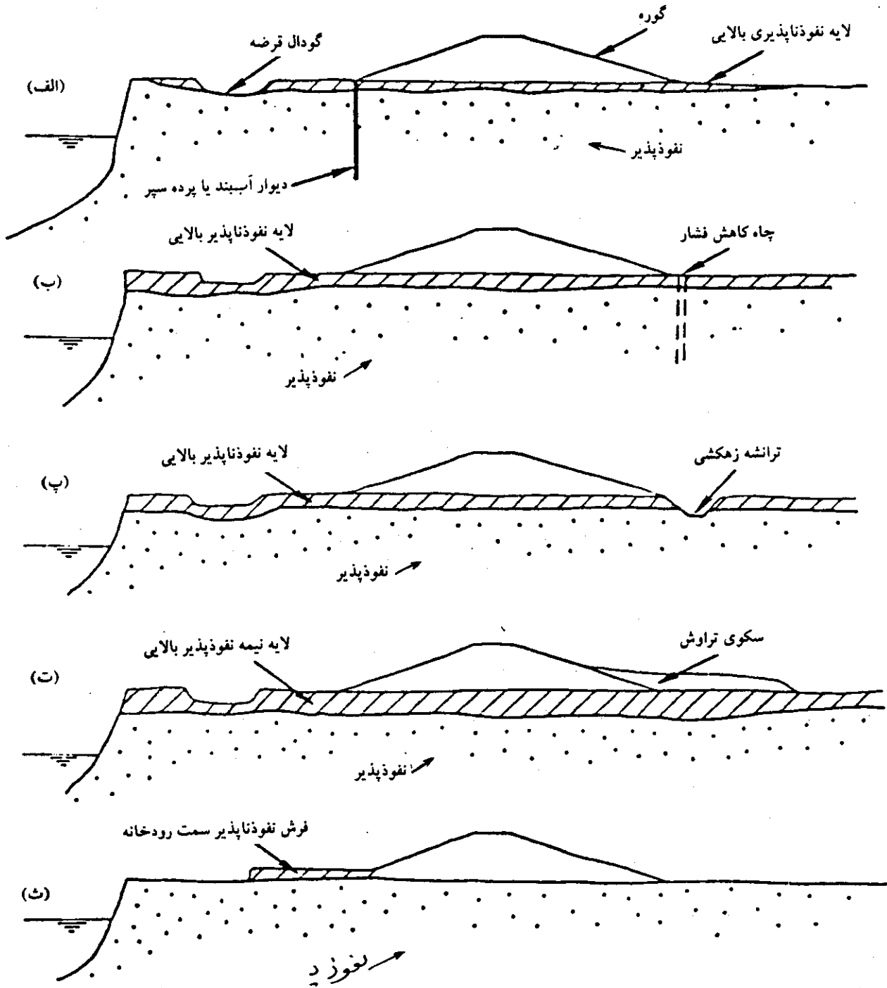
شکل ۴-۳- اقدامات مهار تراوش در زیرگوره‌ها
