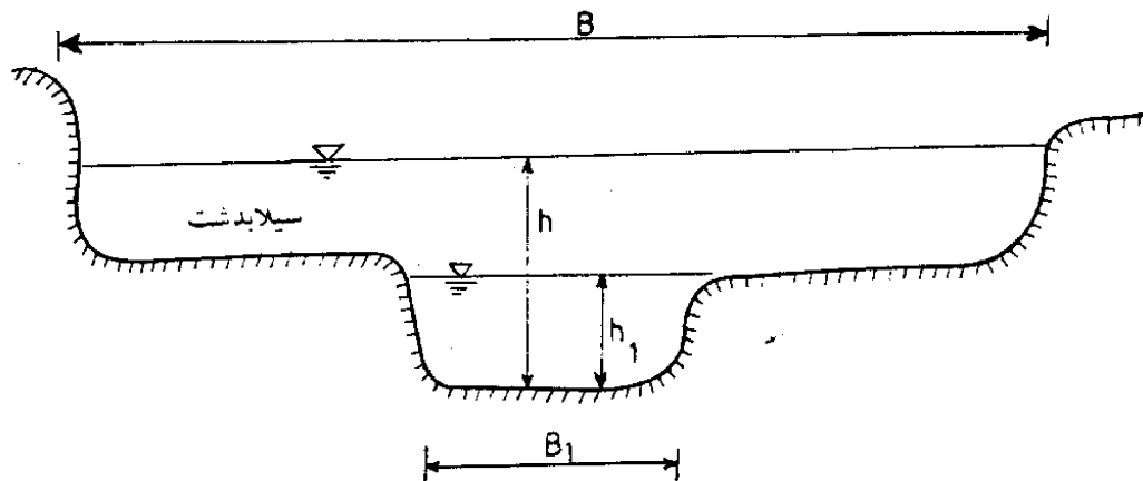
شکل ۳-۶- مقطع رودخانه و سیلابدشت در شرایط سیلابی
