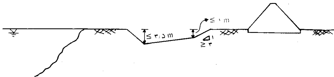
شکل ۳-۸-ب: مقطع عرضی از گوره و محل قرضه در حاشیه رودخانه
