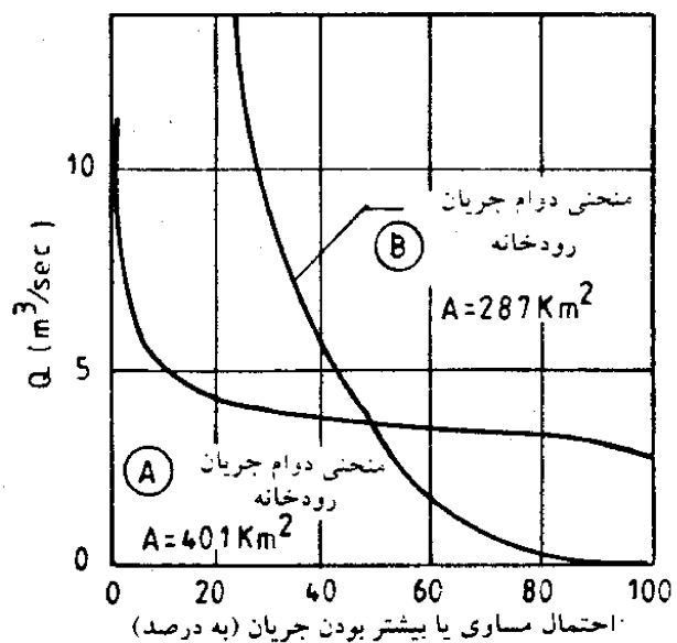
شکل ۳-۴- نمونه‌هایی از منحنی دوام جریان
