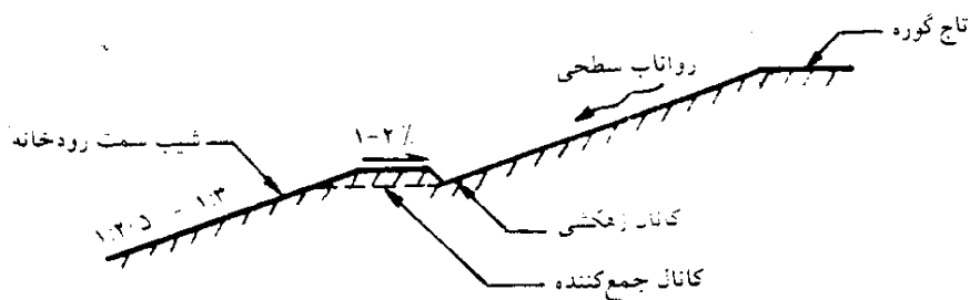
شکل ۱-۴- احداث پله (سکو) همراه با یک کانال زهکشی در طول شیروانی گوره
