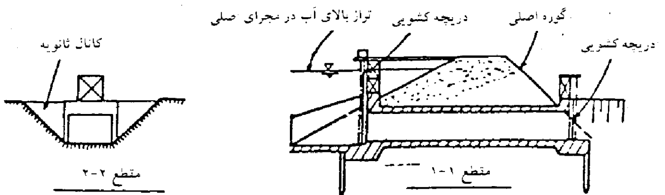
شکل ۴-۱۷- زیرگذر در بدنه گورده (با دریچه های کشویی)
