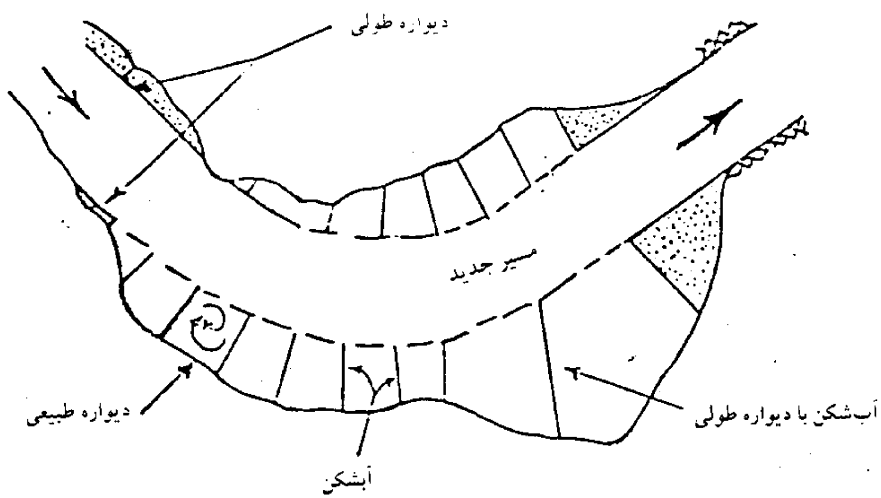
شکل ۴-۱۲- کاربرد آبشکن برای مهار فرسایش و اصلاح مسیر
