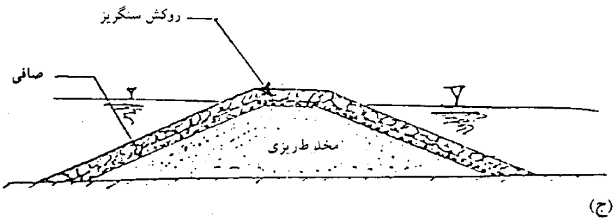
شکل ۴-۱۳- پلان و مقاطع آبشکن نوع سنگریز: الف - پلان، ب - مقطع طولی، ج - مقطع عرضی
