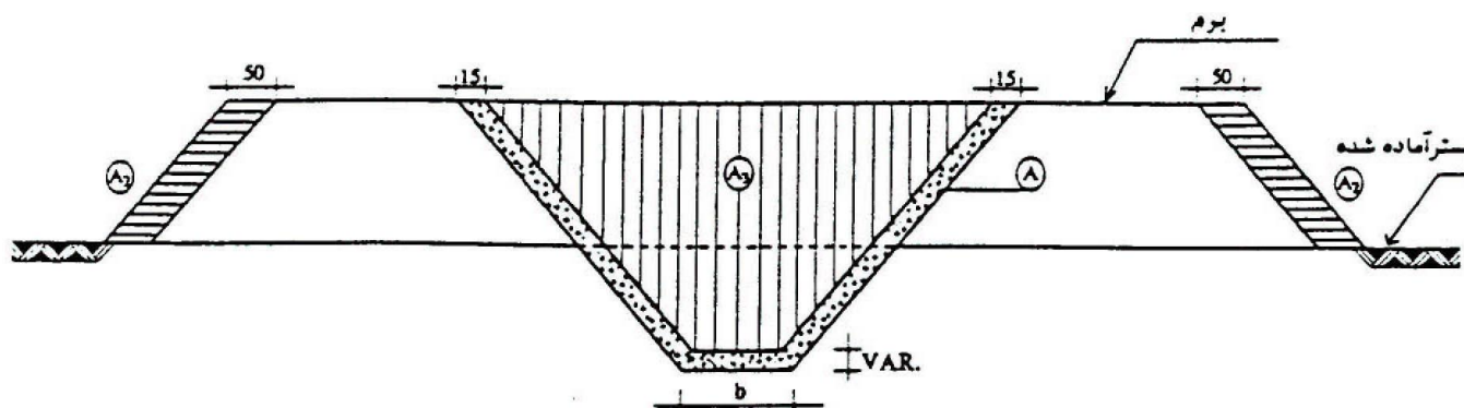
شکل ۶-۳. شمای مقطع خاکبرداری
