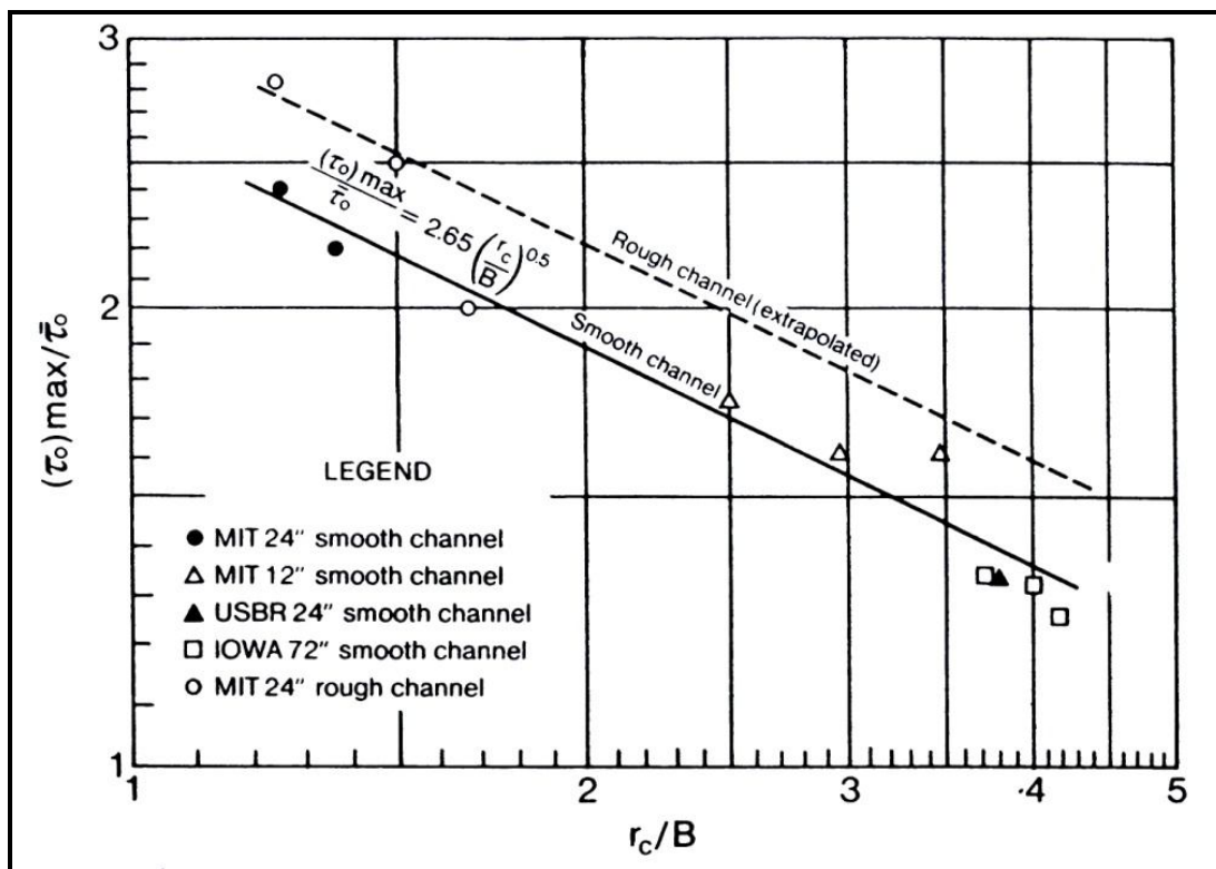
شکل ۳-۳- تنش برشی مرزی بیشینه در پیچانوورها [۵۷]
