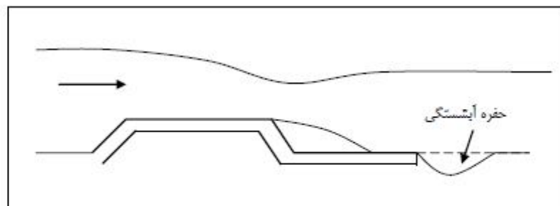
شکل ۸-۶- آبستگي پایین دست آستانه با تاج پهن [۲۶]
