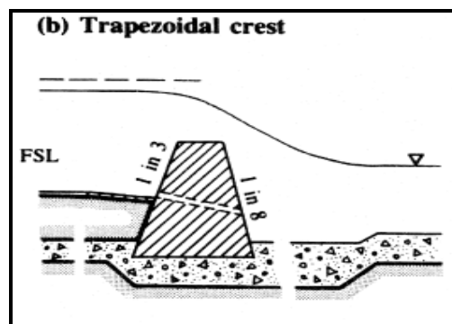
شکل ۹-۱۱- تاج دوزنقه‌ای [۸۶]
