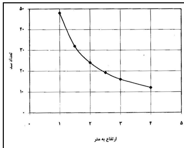
شکل ۶-۱۵- تغییرات تعداد سد نسبت به ارتفاع‌های مختلف آن [۵]
