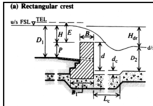
شکل ۹-۱۰- تاج مستطیلی [۸۶]
