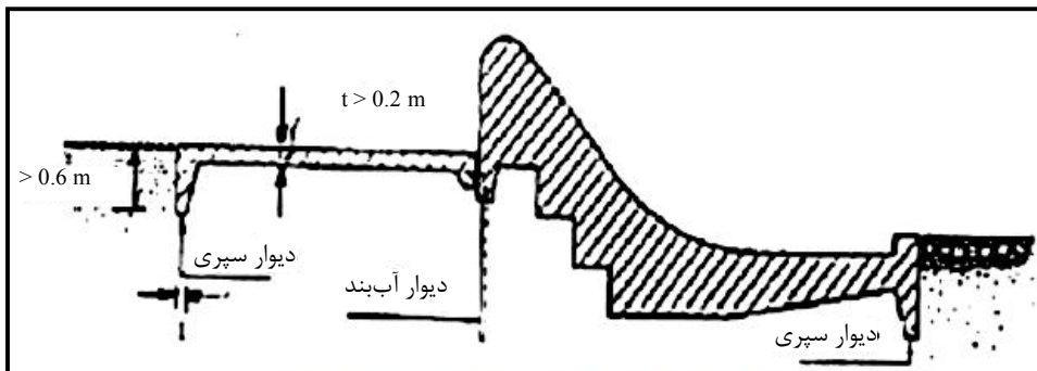
شکل ۹-۴- دیوارهای سپری در بالادست و پایین دست شیب‌شکن‌ها [۲۵]
