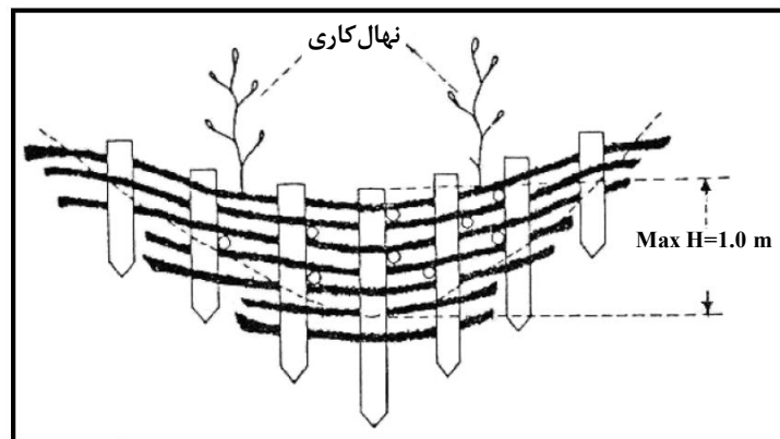
شکل ۱-۴- نمای جلویی سد اصلاحی چپری [۱۳]
