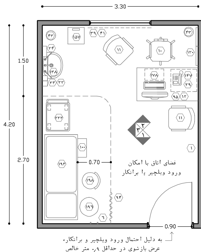
نقشه‌ی ۶۷-۲- پلان نمونه‌ی اتاق معاینه عمومی (چند تخصصی) (برای ۳۰ هزار پذیرش سالیانه) - مقیاس ۱:۵۰
