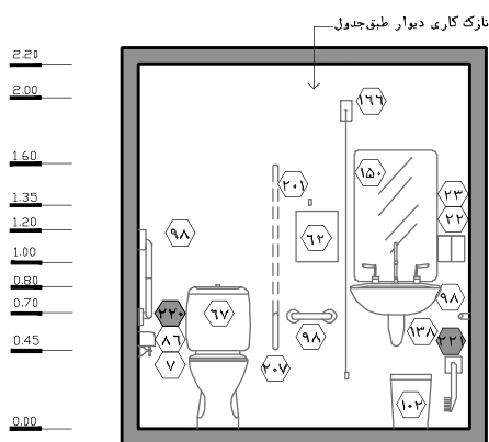
نقشه‌ی ۲-۳۵- نمای ۱ - مقیاس ۱:۵۰
