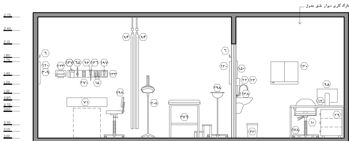
نقشه‌ی ۱۰۷-۲ - نمای ۱ - مقیاس ۱:۵۰
