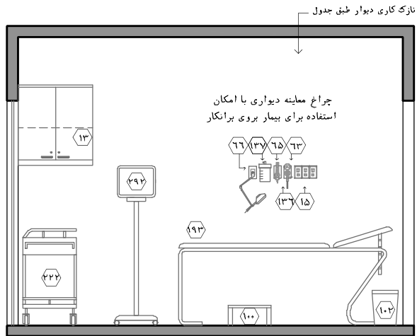
نقشه‌ی ۲-۱۲- نمای ۴- مقیاس ۱:۵۰
