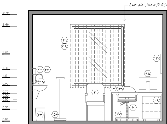
نقشه‌ی ۲-۶۹- نمای ۲- مقیاس ۱:۵۰
