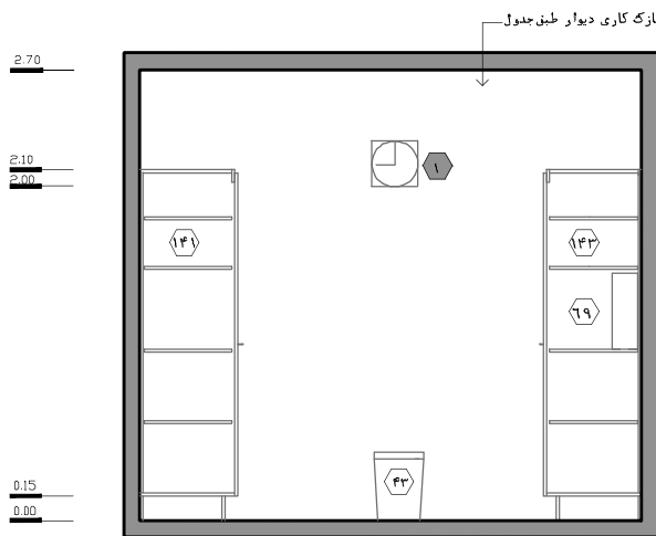
نقشه‌ی ۱۴۴-۲- نمای ۴ - مقیاس ۱:۵۰
