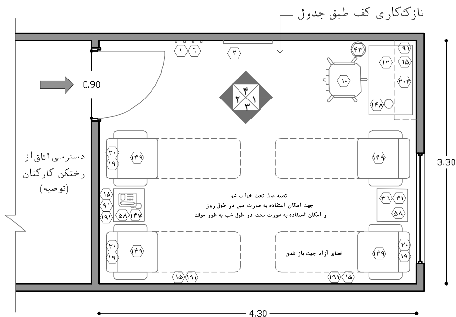
نقشه‌ی ۲-۵۳- پلان نمونه‌ی اتاق استراحت کارکنان (خانم‌ها، آقایان) (برای ۳۰ هزار پذیرش سالیانه) - مقیاس ۱:۵۰
