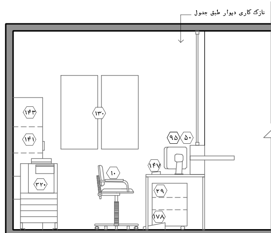
نقشه‌ی ۲-۲۳ - نمای ۳ - مقیاس ۱:۵۰
