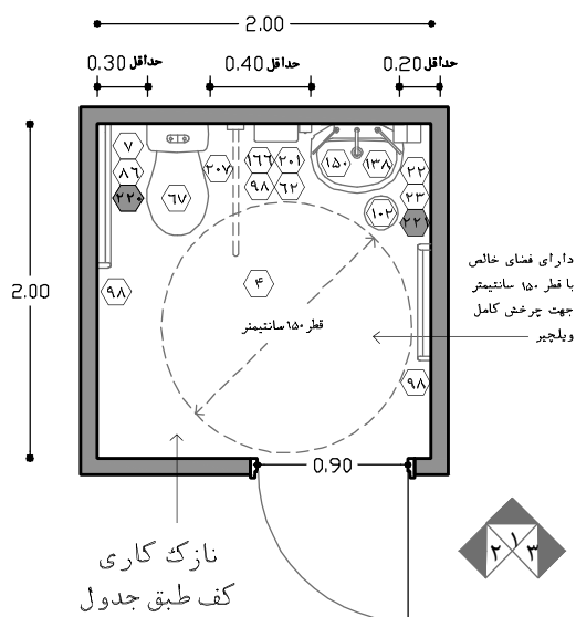
نقشه‌ی ۲-۳۴- پلان نمونه‌ی سرویس بهداشتی معلولین (برای ۳۰ هزار پذیرش سالیانه) - مقیاس ۱:۵۰
