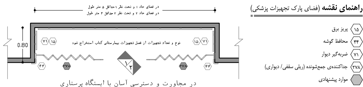
نقشه‌ی ۲-۱۴۵- پلان نمونه‌ی فضای پارک تجهیزات پزشکی حاد ۱ و ۲ (برای ۳۰ هزار پذیرش سالیانه) - مقیاس ۱:۵۰
