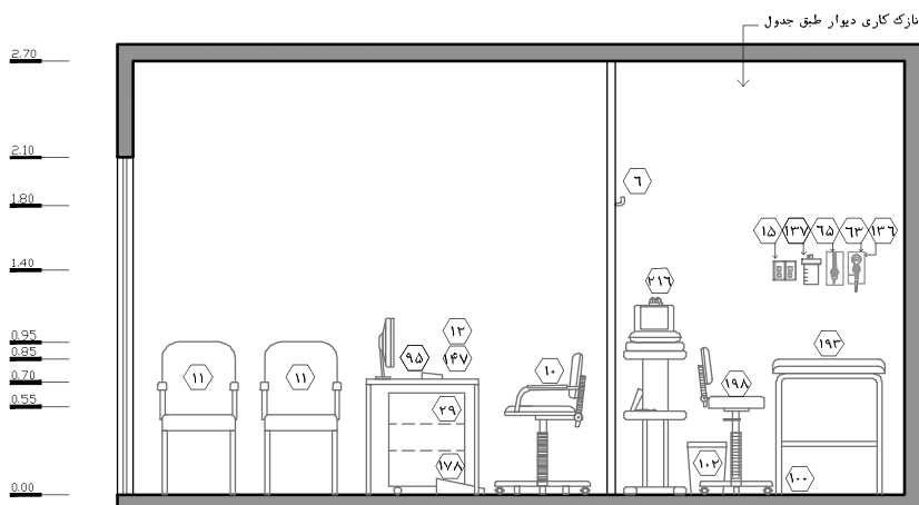
نقشه‌ی ۲-۹۶ نمای ۱ - مقیاس ۱:۵۰
