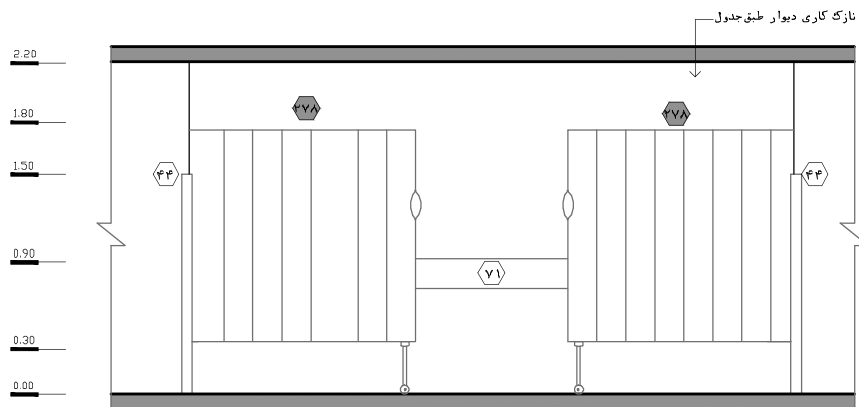
نقشه‌ی ۲-۱۴۶- نمای ۱ - مقیاس ۱:۵۰
