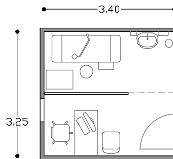
نقشه‌ی ۸۸-۲- اتاق تزریقات و پانسمان با فضای استقرار مسئول اتاق
