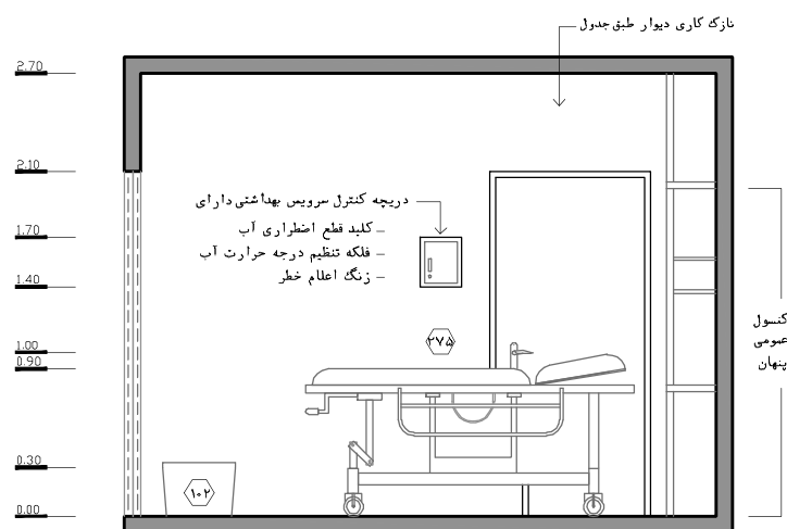
نقشه‌ی ۱۲۶-۲ - نمای ۱ - مقیاس ۱:۵۰
