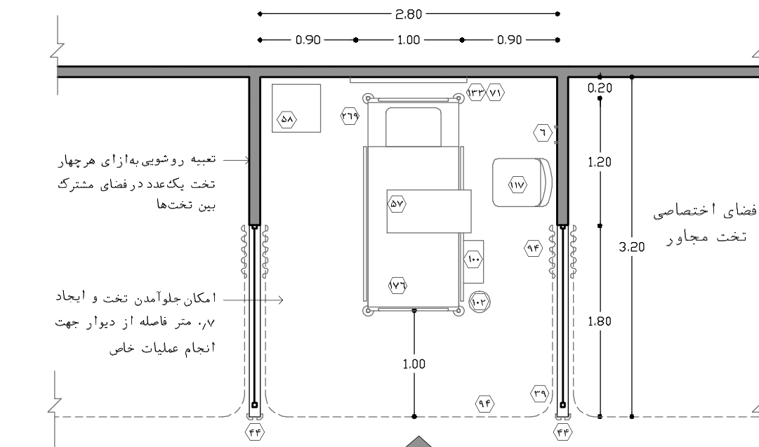
نقشه‌ی ۲-۱۷۸ - پلان نمونه‌ی فضای بستری تحت نظر سطح ۲ (برای ۳۰ هزار پذیرش سالانه) - مقیاس ۱:۵۰
