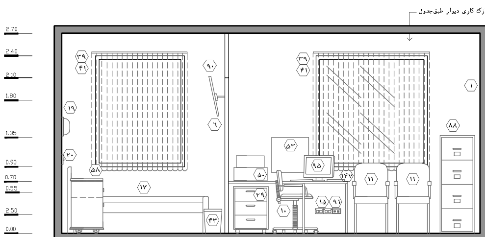
نقشه‌ی ۲-۵۲-۳ - نمای ۳ - مقیاس ۱:۵۰
