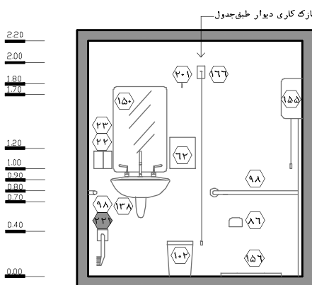
نقشه‌ی ۳۳-۲- نمای ۱ - مقیاس ۱:۵۰
