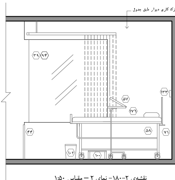
نقشه‌ی ۲-۱۸۰ - نمای ۲ - مقیاس ۱:۵۰
