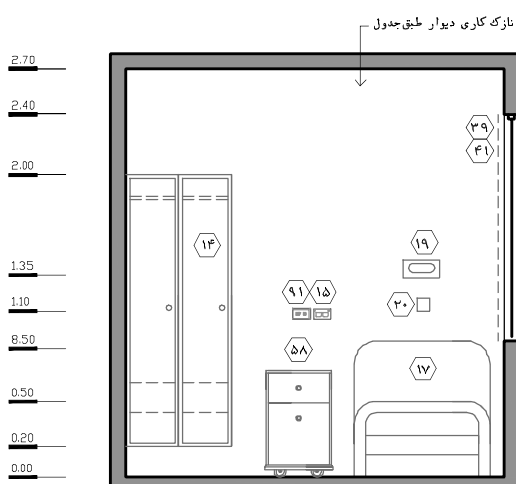
نقشه‌ی ۲-۵۱-۲ - نمای ۲ - مقیاس ۱:۵۰
