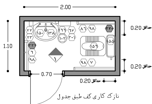
نقشه‌ی ۳۲-۲- پلان نمونه‌ی سرویس بهداشتی عمومی (برای ۳۰ هزار پذیرش سالیانه) - مقیاس ۱:۵۰
