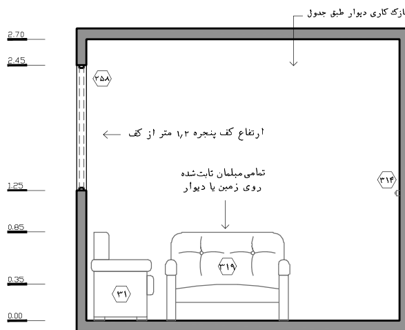
نقشه‌ی ۲-۸۱- نمای ۲ - مقیاس ۱:۵۰
