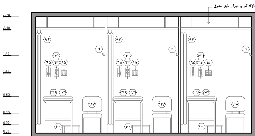
نقشه‌ی ۲-۸۳- نمای ۱ - مقیاس ۱:۵۰
