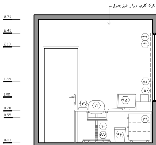
نقشه‌ی ۲-۵۰-۱ - نمای ۱ - مقیاس ۱:۵۰
