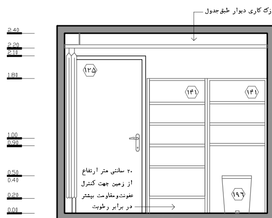
نقشه‌ی ۲-۴۶- نمای ۴ - مقیاس ۱:۵۰
