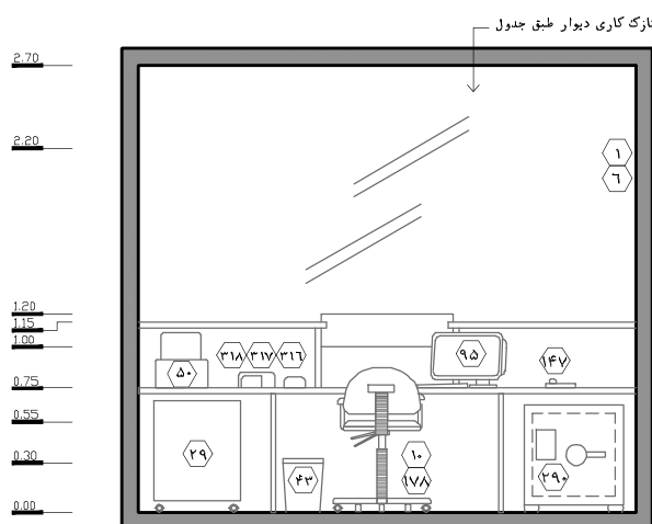
نقشه‌ی ۲-۲۵ - نمای ۱ - مقیاس ۱:۵۰
