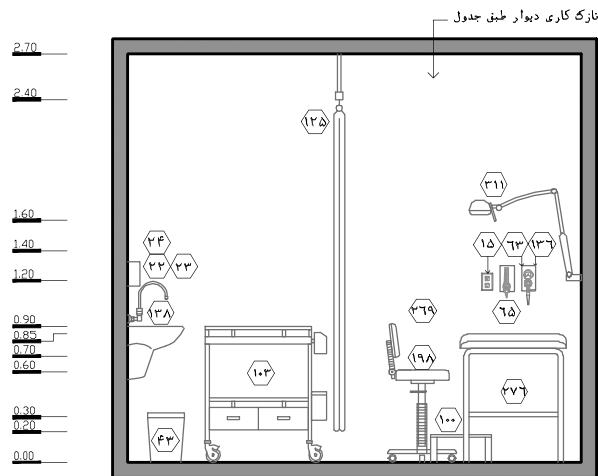
نقشه ۲-۹۴ - نمای ۳ - مقیاس ۱:۵۰
