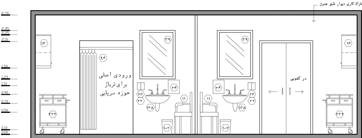
نقشه‌ی ۲-۱۰- نمای ۲- مقیاس ۱:۵۰
