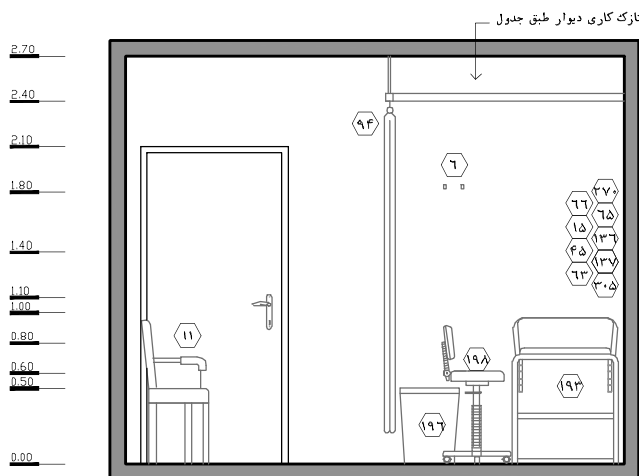
نقشه‌ی ۲-۶۸- نمای ۱- مقیاس ۱:۵۰
