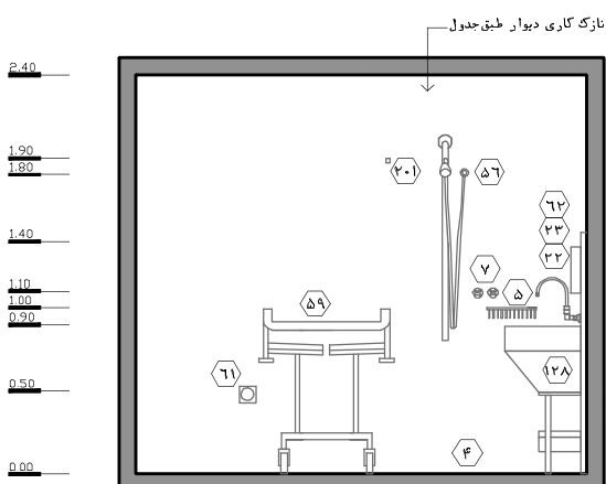
نقشه‌ی ۲-۴۵- نمای ۳ - مقیاس ۱:۵۰
