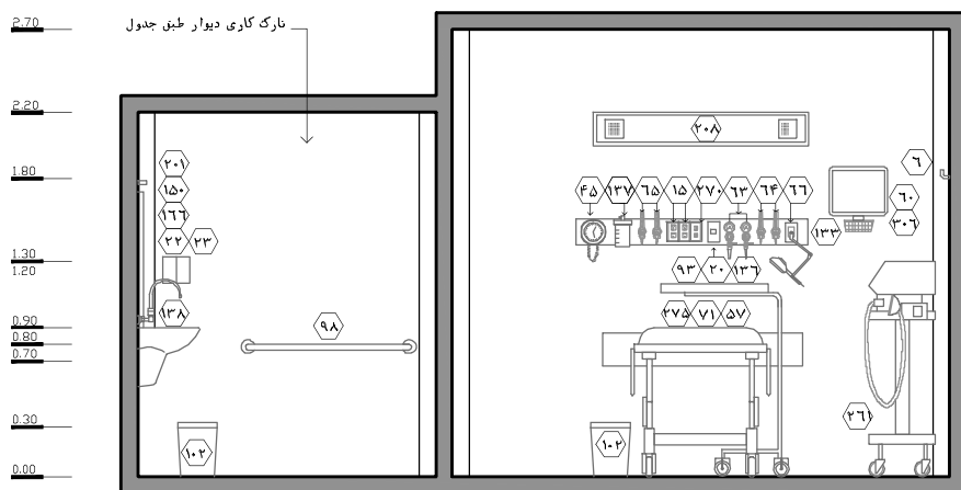
نقشه‌ی ۲-۱۳۳-۲ - نمای ۲ - مقیاس ۱:۵۰
