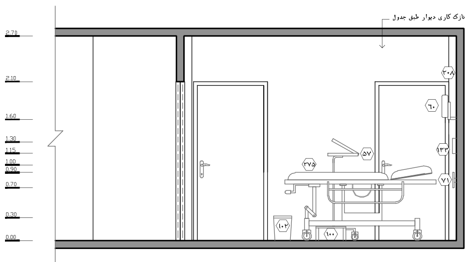
نقشه‌ی ۳-۱۳۴-۲ - نمای ۳ - مقیاس ۱:۵۰
