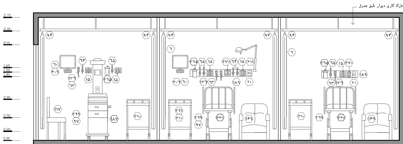
نقشه‌ی ۱-۲-۱۲۱- نمای ۱ - مقیاس ۱:۵۰
