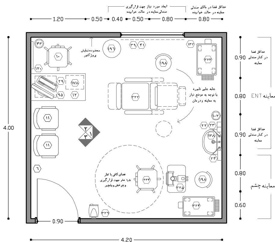
نقشه‌ی ۲-۷۱- پلان نمونه‌ی اتاق معاینه گوش، حلق، بینی/چشم (برای ۳۰ هزار پذیرش سالیانه) - مقیاس ۱:۵۰
