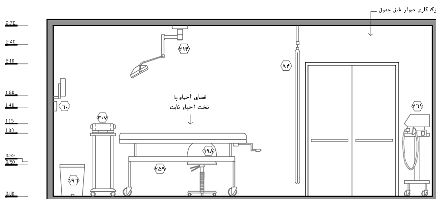
نقشه‌ی ۲-۱۰۲- نمای ۱- مقیاس ۱:۵۰
