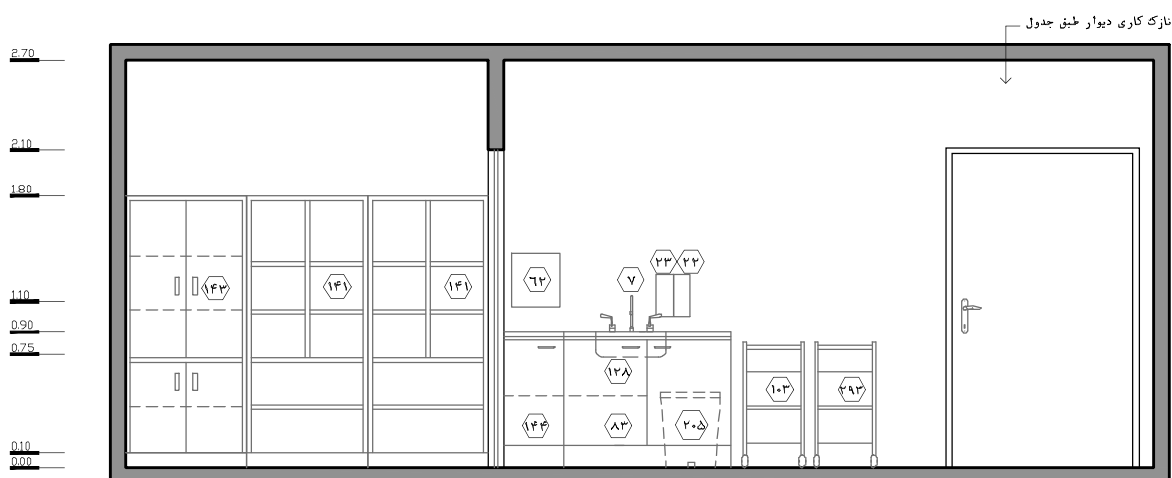
نقشه‌ی ۱۰۹-۲ - نمای ۳ - مقیاس ۱:۵۰
