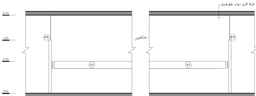
نقشه‌ی ۲-۲- نمای ۱ - مقیاس ۱:۵۰
