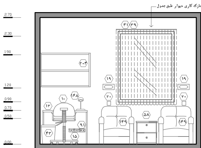
نقشه‌ی ۲-۵۴- نمای ۱ - مقیاس ۱:۵۰
