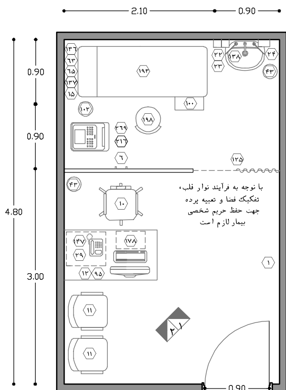
نقشه‌ی ۲-۹۵ پلان نمونه‌ی اتاق نوار قلب (برای ۳۰ هزار پذیرش سالیانه) مقیاس ۱:۵۰
