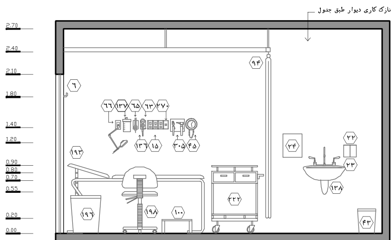
نقشه‌ی ۲-۷۰- نمای ۳- مقیاس ۱:۵۰
