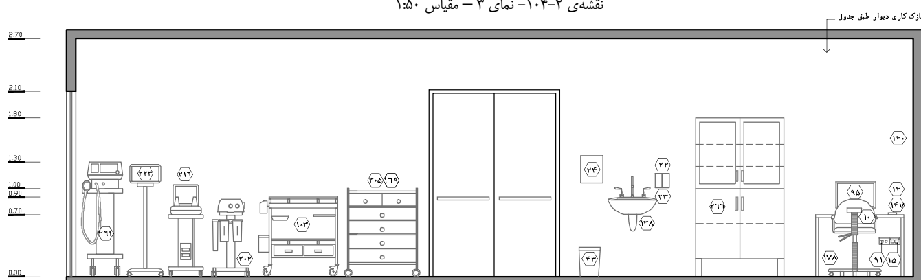
نقشه‌ی ۲-۱۰۵- نمای ۴- مقیاس ۱:۵۰
