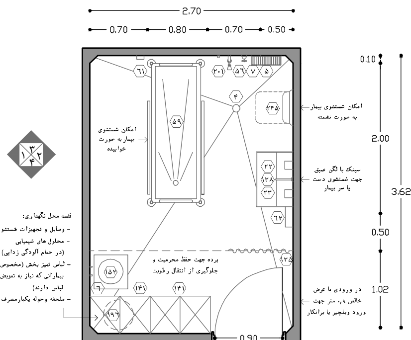
نقشه‌ی ۲-۴۲- پلان نمونه‌ی حمام آلودگی‌زدایی (برای ۳۰ هزار پذیرش سالانه) - مقیاس ۱:۵۰
