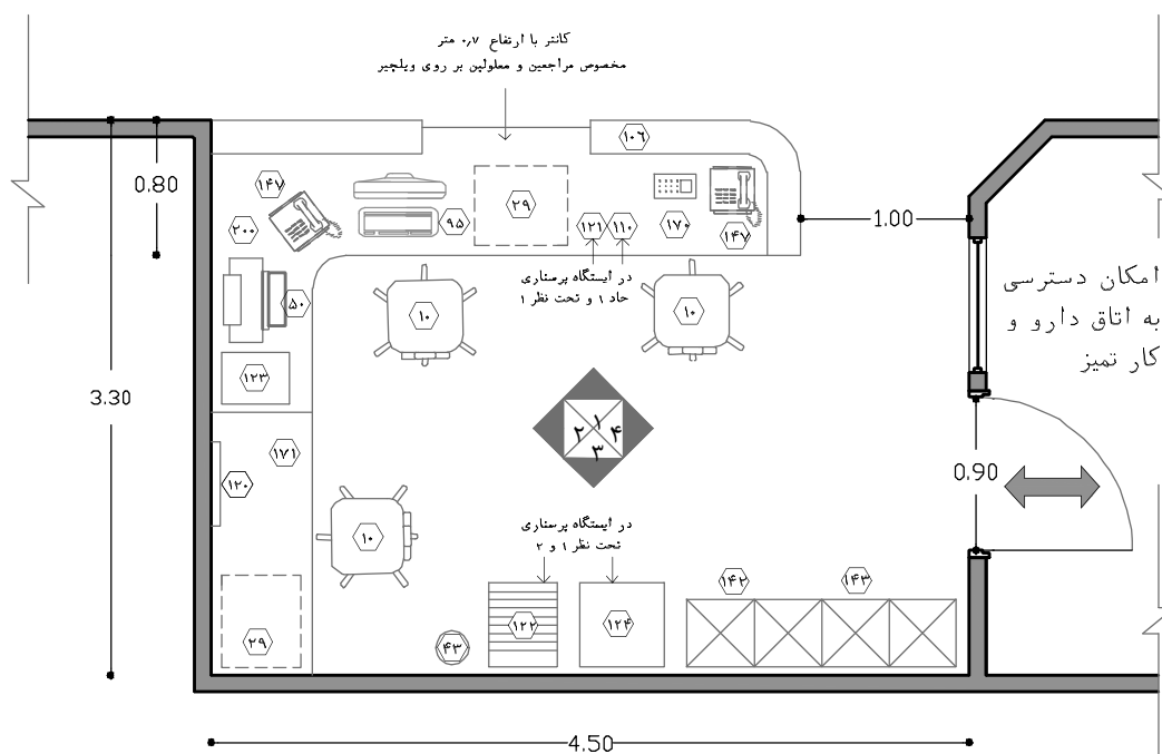
نقشه ۲-۱۳۵- پلان نمونه ایستگاه پرستاری حاد ۲و۱
