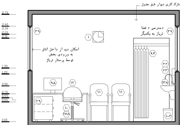
نقشه‌ی ۲-۱۱- نمای ۳- مقیاس ۱:۵۰
