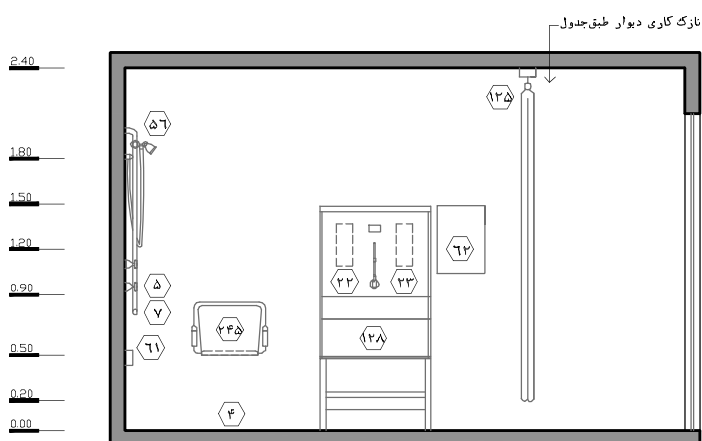
نقشه‌ی ۲-۴۴- نمای ۲ - مقیاس ۱:۵۰
