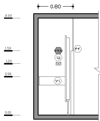
نقشه‌ی ۲-۱۴۷- نمای ۲ - مقیاس ۱:۵۰
