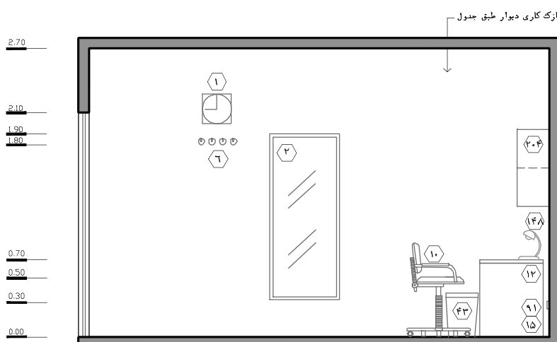
نقشه ۲-۵۷ - نمای ۴ - مقیاس ۱:۵۰
