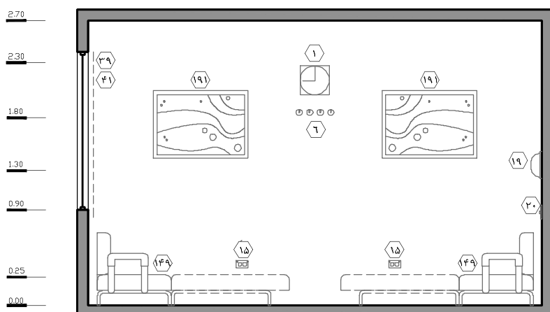
نقشه ۲-۵۶ - نمای ۳ - مقیاس ۱:۵۰
