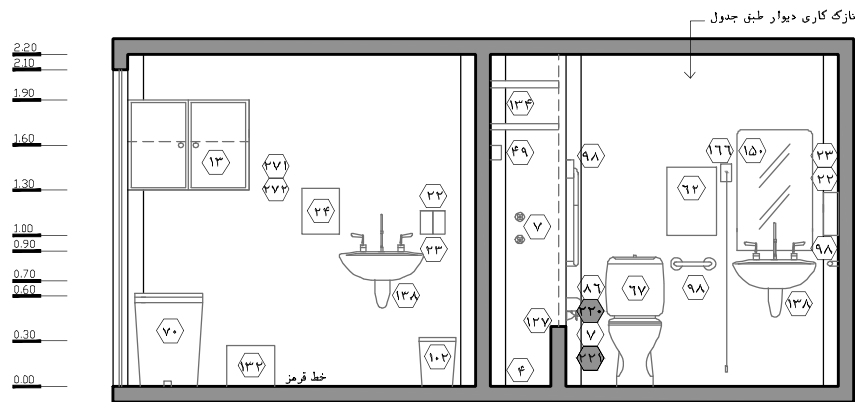
نقشه‌ی ۱-۳۲-۲ - نمای ۱ - مقیاس ۱:۵۰
