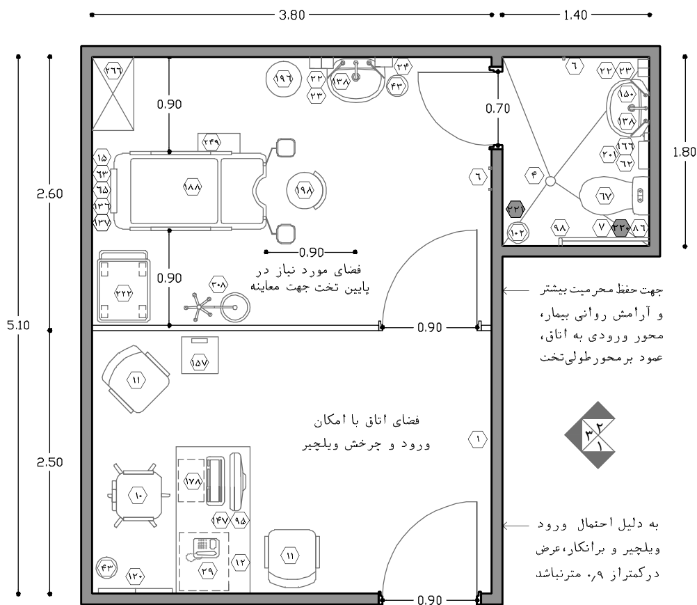
نقشه‌ی ۲-۷۵- پلان نمونه‌ی اتاق معاینه زنان (برای ۳۰ هزار پذیرش سالیانه) - مقیاس ۱:۵۰
