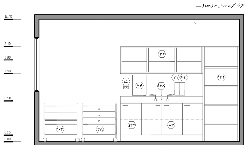
نقشه‌ی ۱۴۱-۲- نمای ۱ - مقیاس ۱:۵۰
