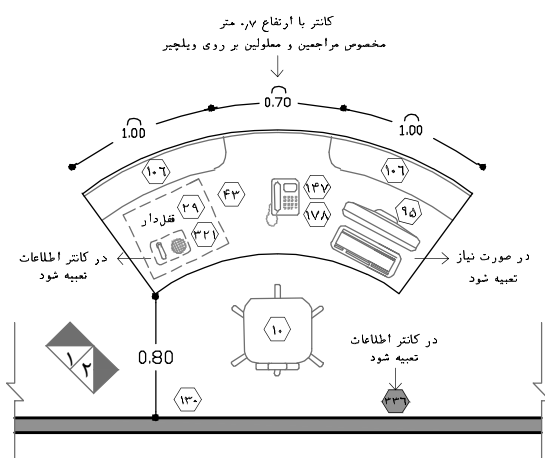
نقشه‌ی ۱۳-۲ - پلان نمونه‌ی اطلاعات / نگهداری / پلیس / کنترل (برای ۳۰ هزار پذیرش سالیانه) - مقیاس ۱:۵۰
