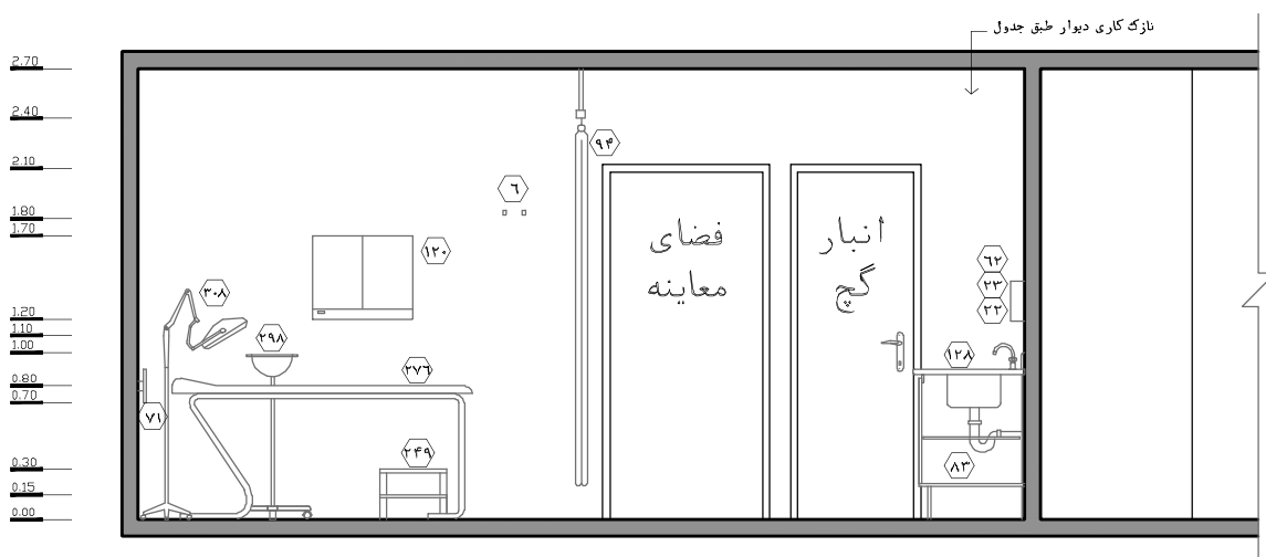
نقشه‌ی ۱۰۸-۲ - نمای ۲ - مقیاس ۱:۵۰
