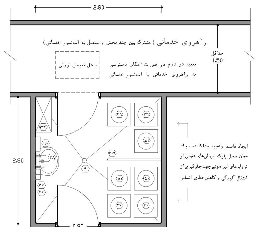
نقشه‌ی ۲-۱۷۲- پلان نمونه‌ی اتاق جمع‌آوری زباله و رخت کثیف (برای ۳۰ هزار پذیرش سالیانه) مقیاس ۱:۵۰
