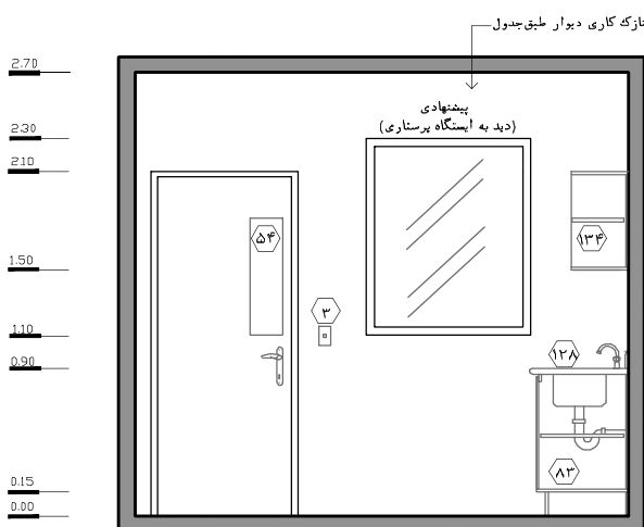
نقشه‌ی ۱۴۳-۲- نمای ۳ - مقیاس ۱:۵۰
