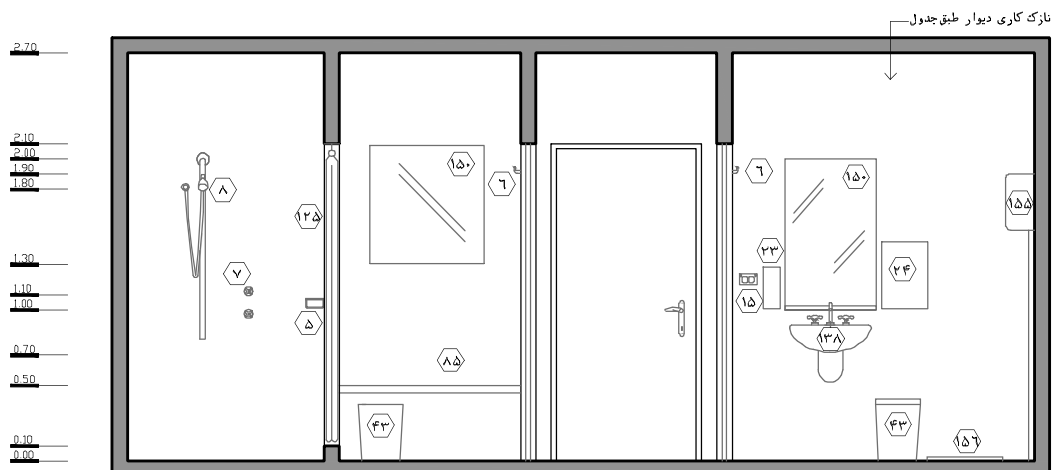
نقشه‌ی ۲-۶۱- نمای ۳- مقیاس ۱:۵۰
