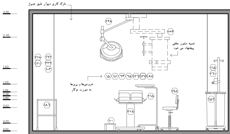
نقشه‌ی ۲-۱۱۱- نمای ۱- مقیاس ۱:۵۰
