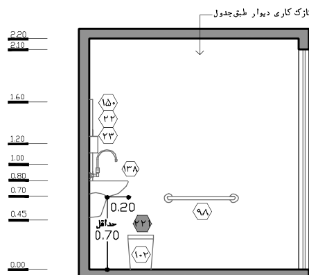
نقشه‌ی ۲-۳۷- نمای ۳ - مقیاس ۱:۵۰
