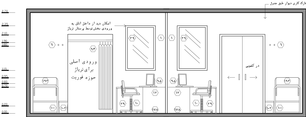
نقشه‌ی ۹-۲- نمای ۱- مقیاس ۱:۵۰
