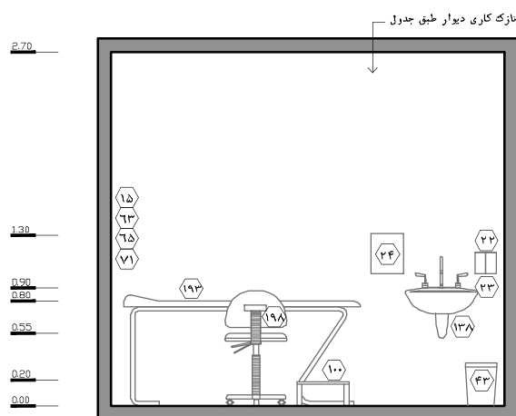
نقشه‌ی ۲-۹۶ نمای ۱ - مقیاس ۱:۵۰
