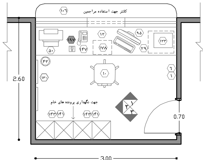
نقشه‌ی ۲-۱۶- پلان نمونه‌ی کانتر/کابین پذیرش (برای ۳۰ هزار پذیرش سالیانه) - مقیاس ۱:۵۰
