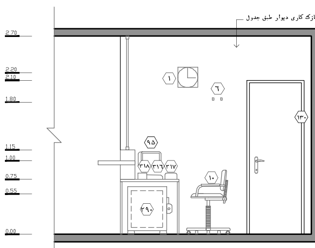
نقشه‌ی ۲-۲۶ - نمای ۲ - مقیاس ۱:۵۰
