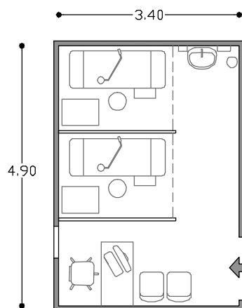
نقشه‌ی ۹۰-۲- اتاق تزریقات و پانسمان دو تختی با فضای استقرار مسئول اتاق
