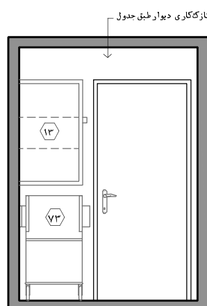
نقشه‌ی ۱۶۰-۲ - نمای ۲ - مقیاس ۱:۵۰
