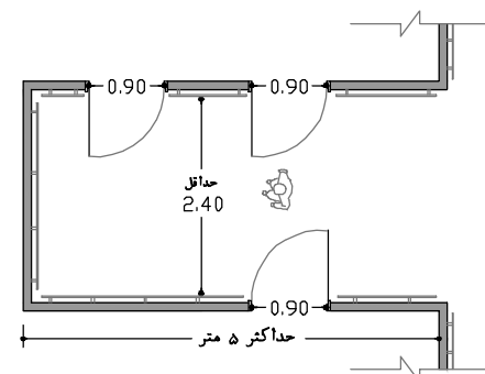
نقشه ۲-۱۹۱- راهرو با عرض حداقل ۲/۴ متر مقیاس ۱:۱۰۰
