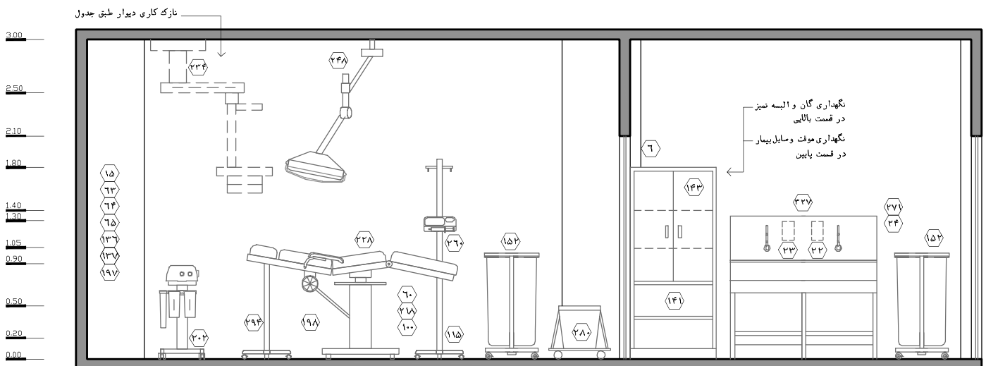
نقشه‌ی ۲-۱۱۲- نمای ۲- مقیاس ۱:۵۰
