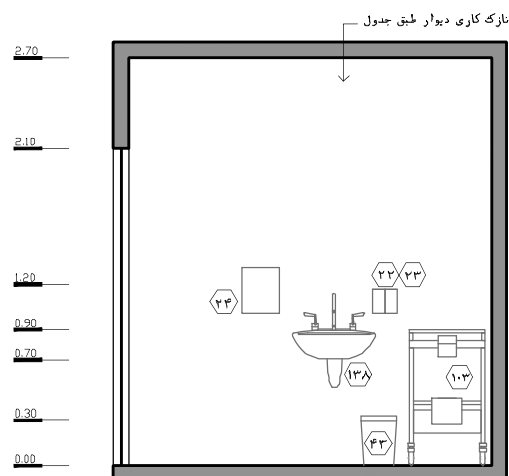
نقشه ۲-۹۳ - نمای ۲ - مقیاس ۱:۵۰
