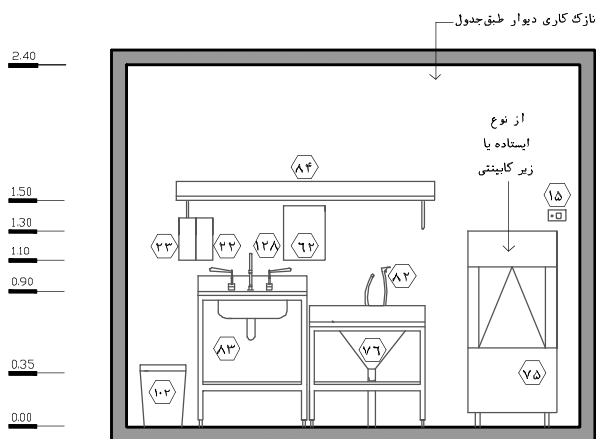
نقشه‌ی ۲-۱۶۹- نمای ۱ - مقیاس ۱:۵۰
