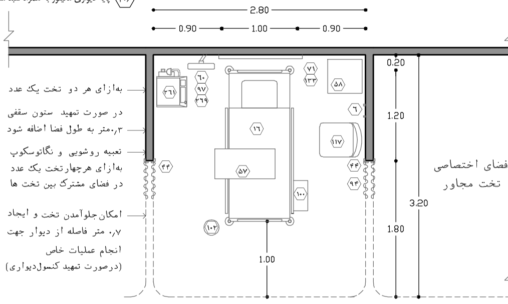
نقشه ۲-۱۷۵-۲ پلان نمونه‌ی فضای بستری
