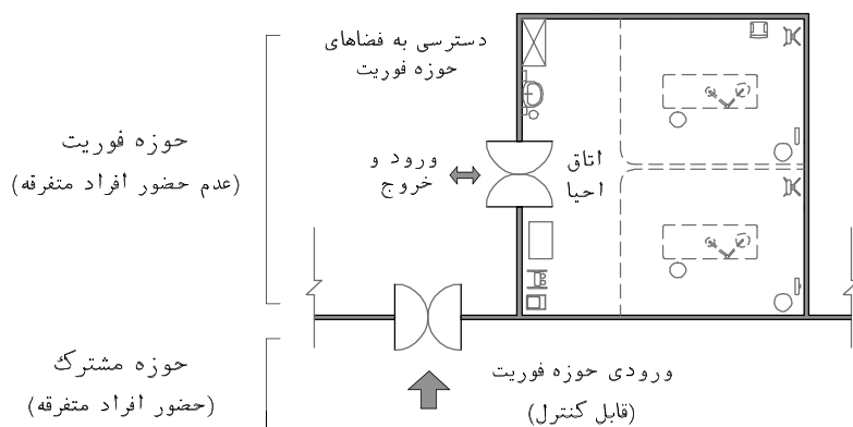
نقشه‌ی شماری ۹۸-۲- اتاق احیا دارای یک در
