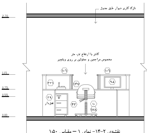
نقشه‌ی ۱۴-۲ - نمای ۱ - مقیاس ۱:۵۰
