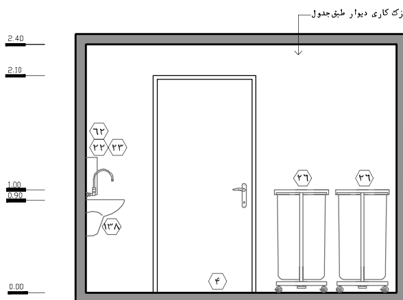
نقشه‌ی ۱۷۴-۲ - نمای ۲ - مقیاس ۱:۵۰
