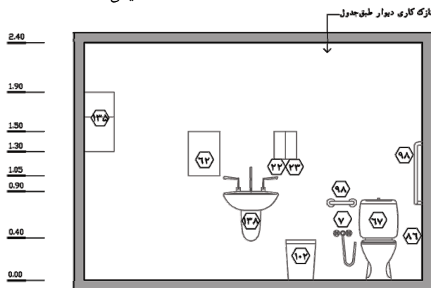
نما ۲- مقیاس : ۱:۵۰
