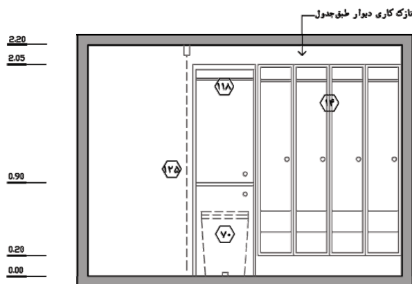
نما ۱ - مقیاس : ۱:۵۰
