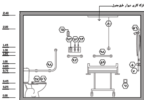
نما ۳- مقیاس : ۱:۵۰
