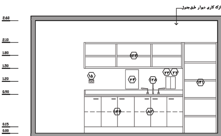
نما ۲ - مقیاس : ۱:۵۰
