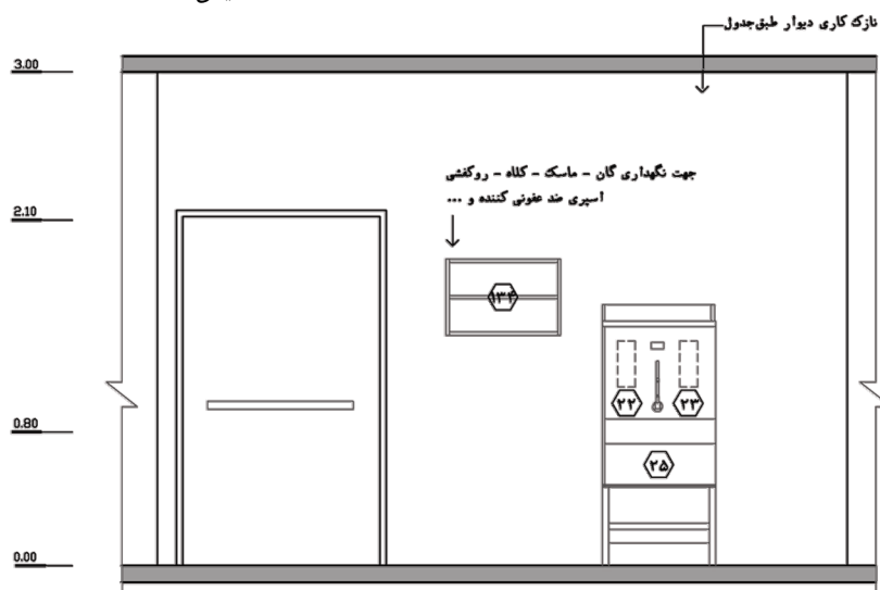
نما ۴- مقیاس : ۱:۵۰
