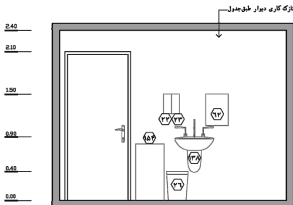
نما ۲ - مقیاس : ۱:۵۰
