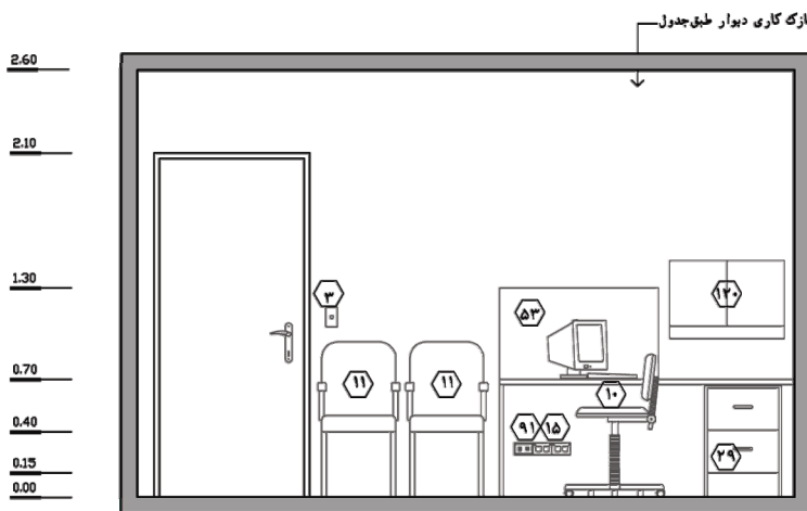
نما ۱ - مقیاس : ۱:۵۰
