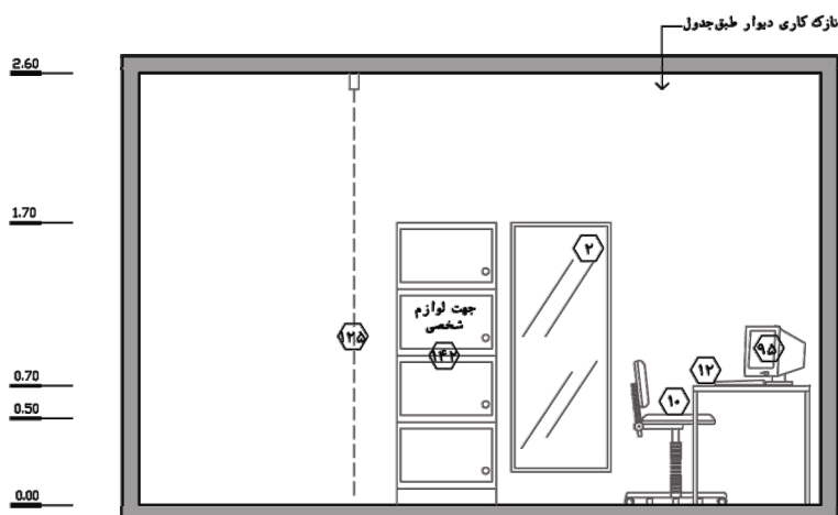
نما ۲ - مقیاس : ۱:۵۰
