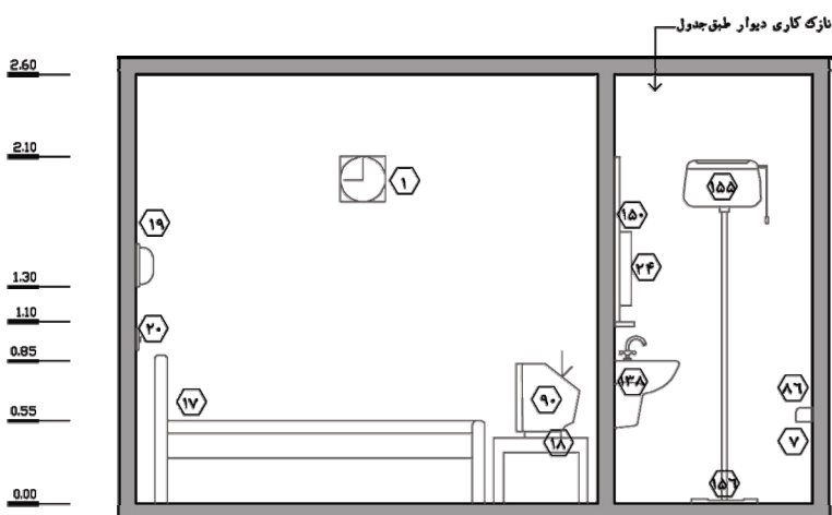
نما ۳ - مقیاس : ۱:۵۰
