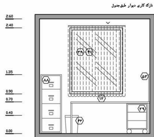
نما ۲ - مقیاس : ۱:۵۰
